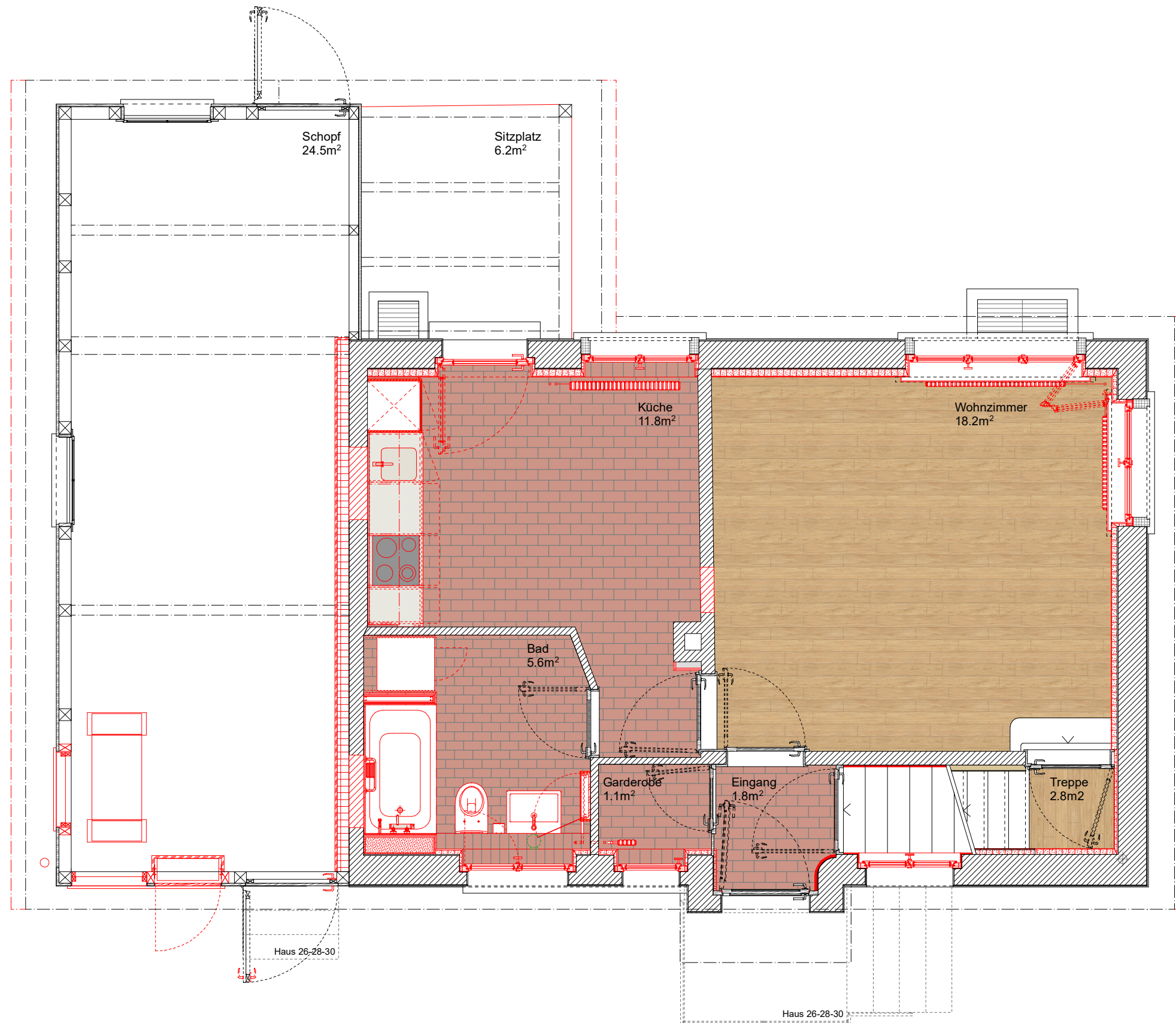
Grundriss Erdgeschoss
