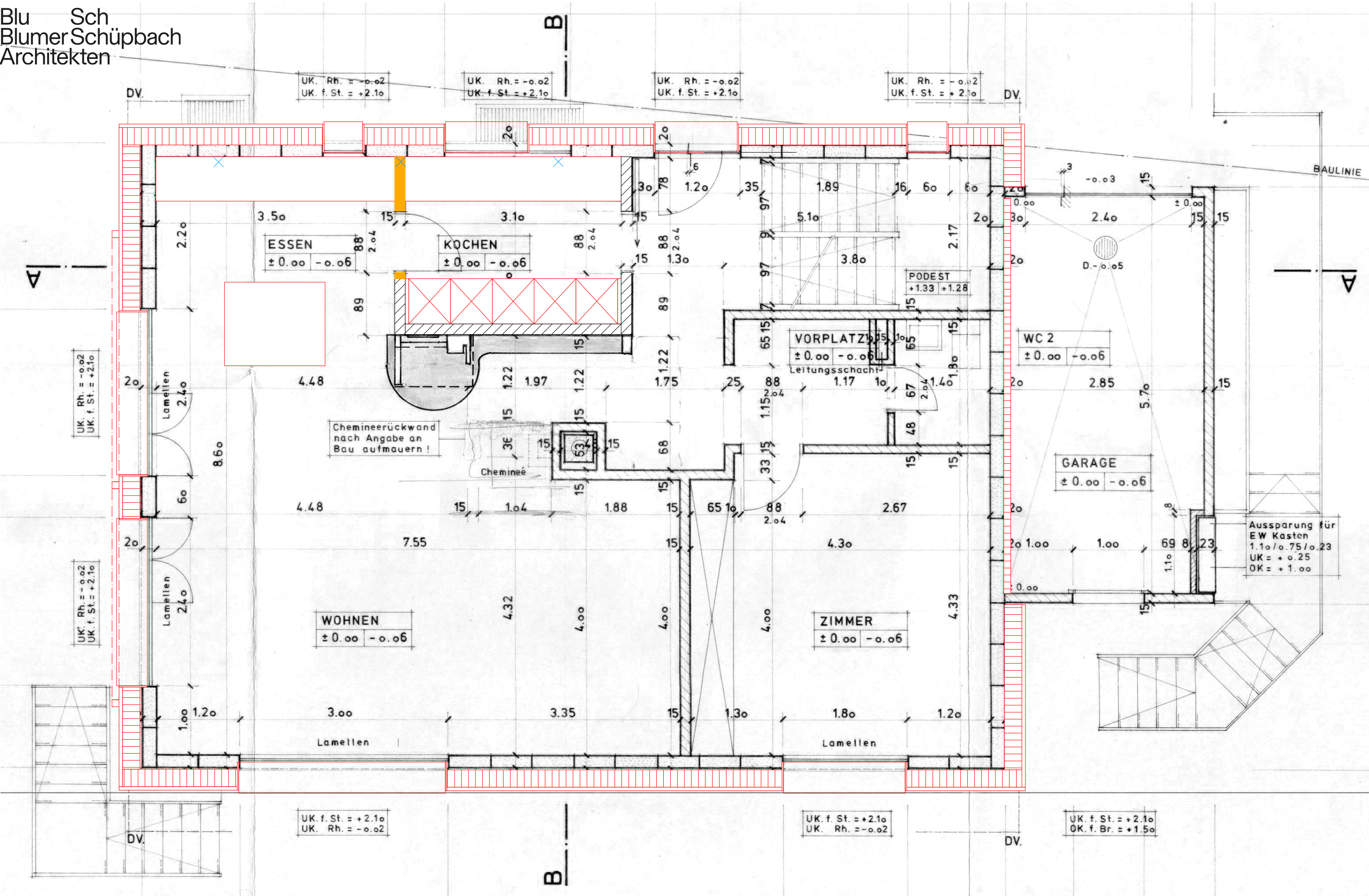
Grundriss Erdgeschoss
