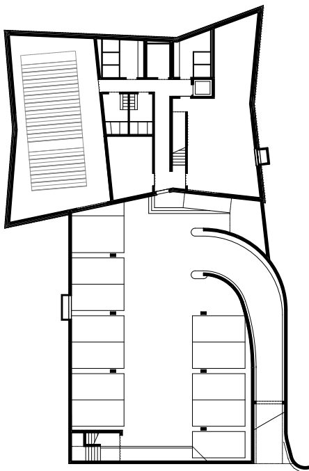
Grundriss 1.Untergeschoss M1:500
