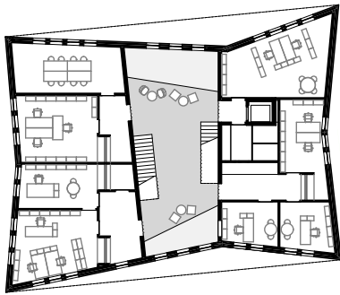
Grundriss 1.Obergeschoss M1:500
