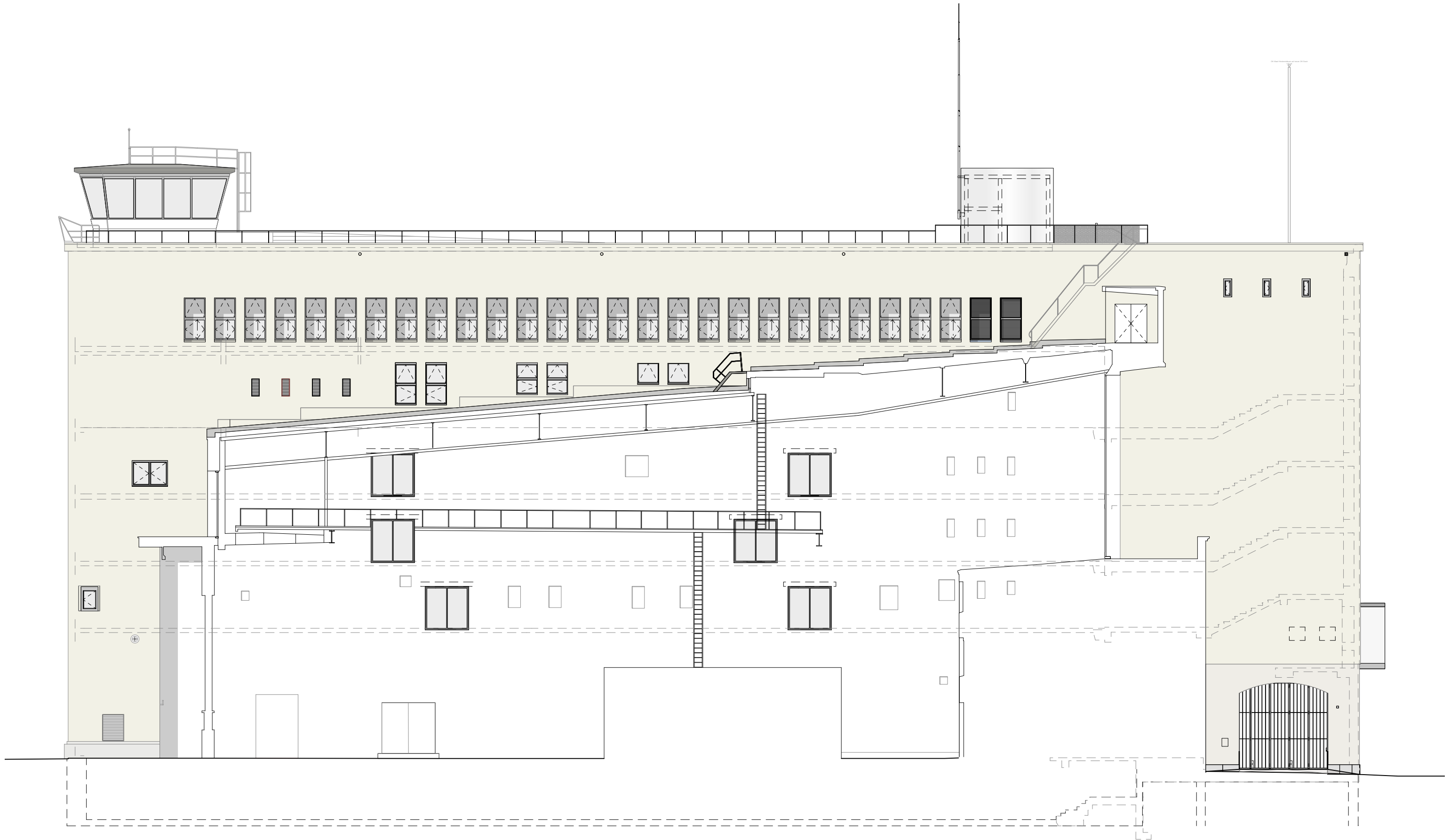
THF - Ansicht Nord
