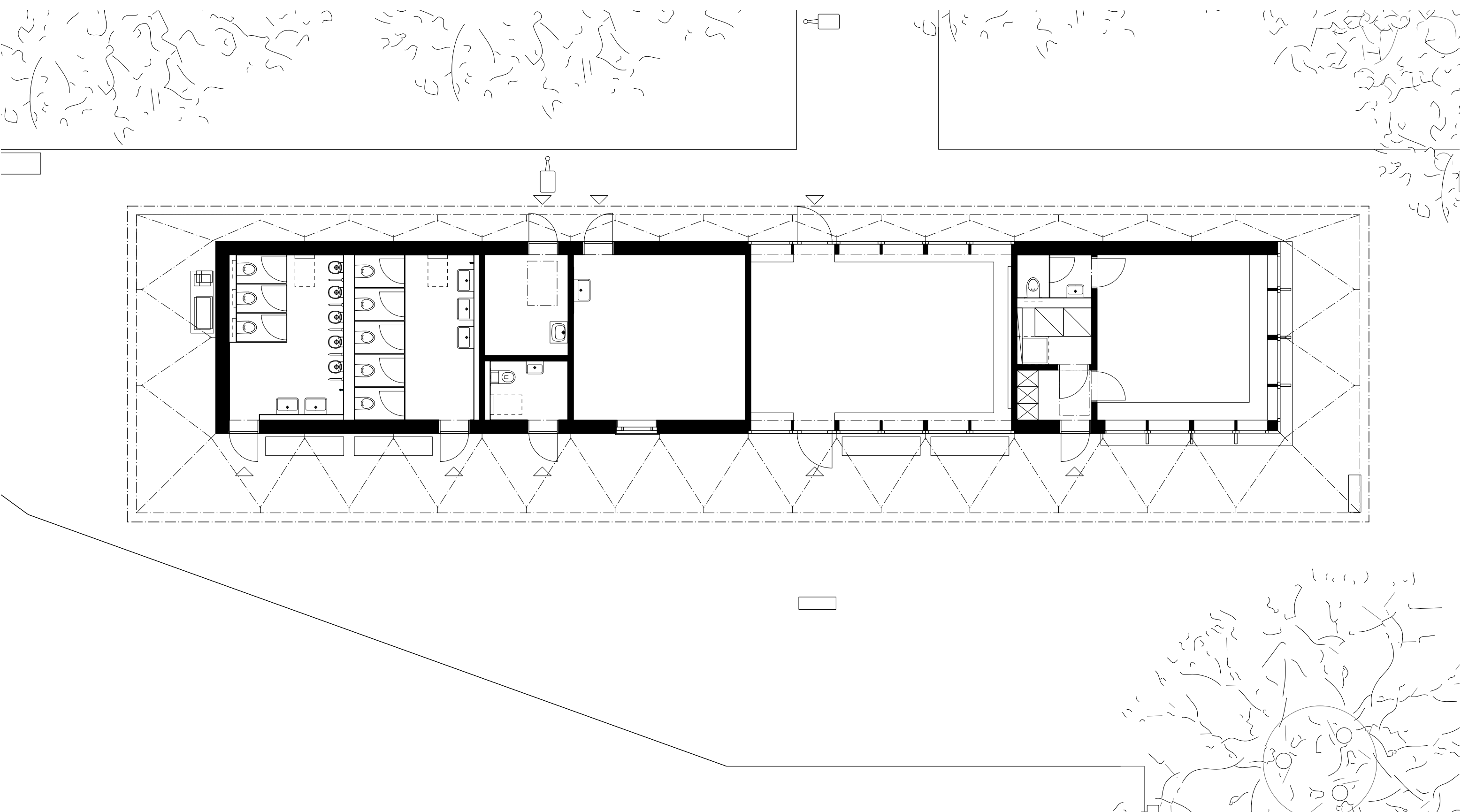
GRUNDRISS ERDGESCHOSS
