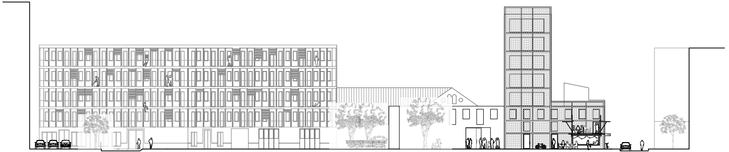
SCHNITT A 1:200
