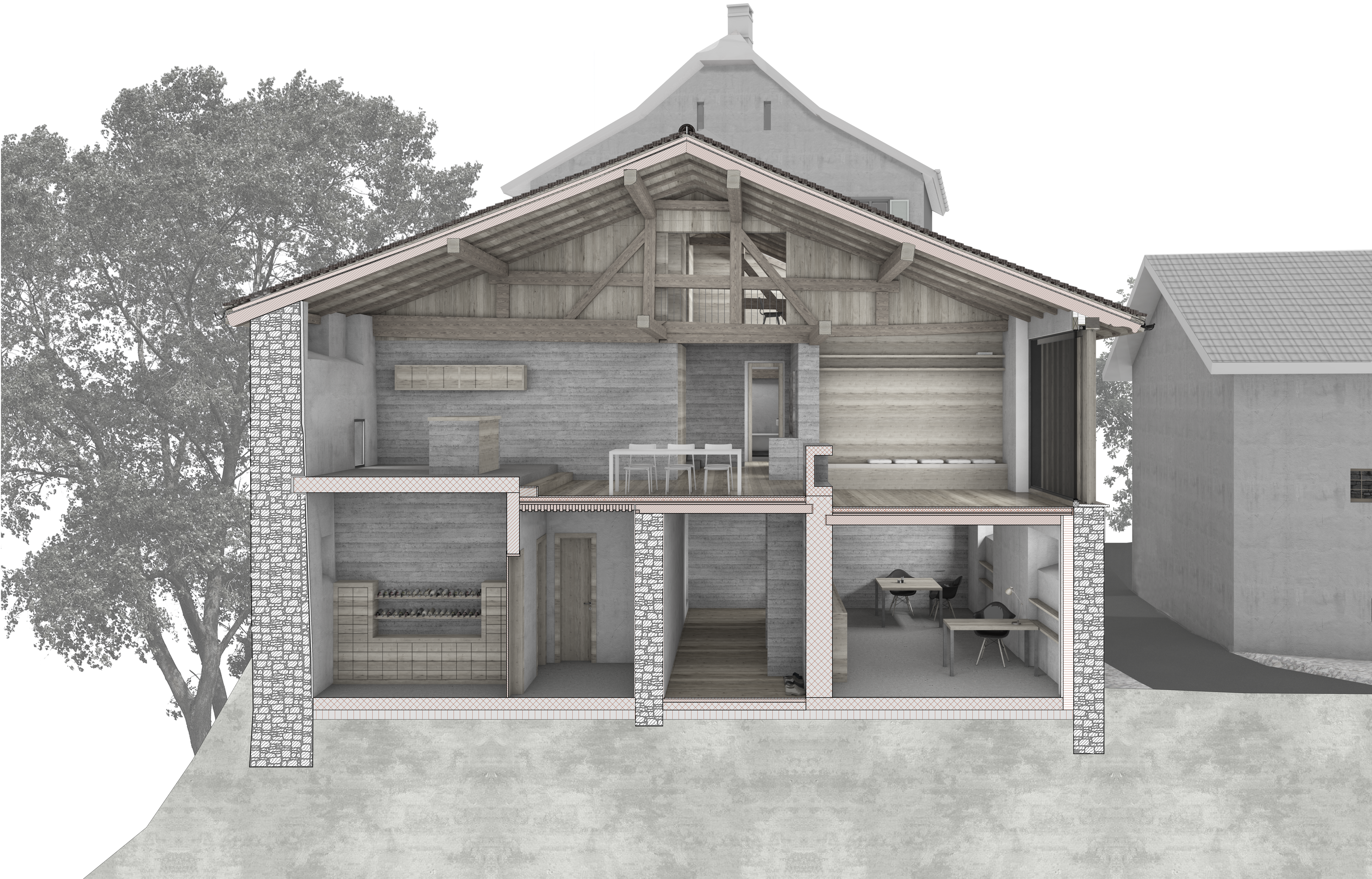
SCHNITTVISUALISIERUNG 1:20
