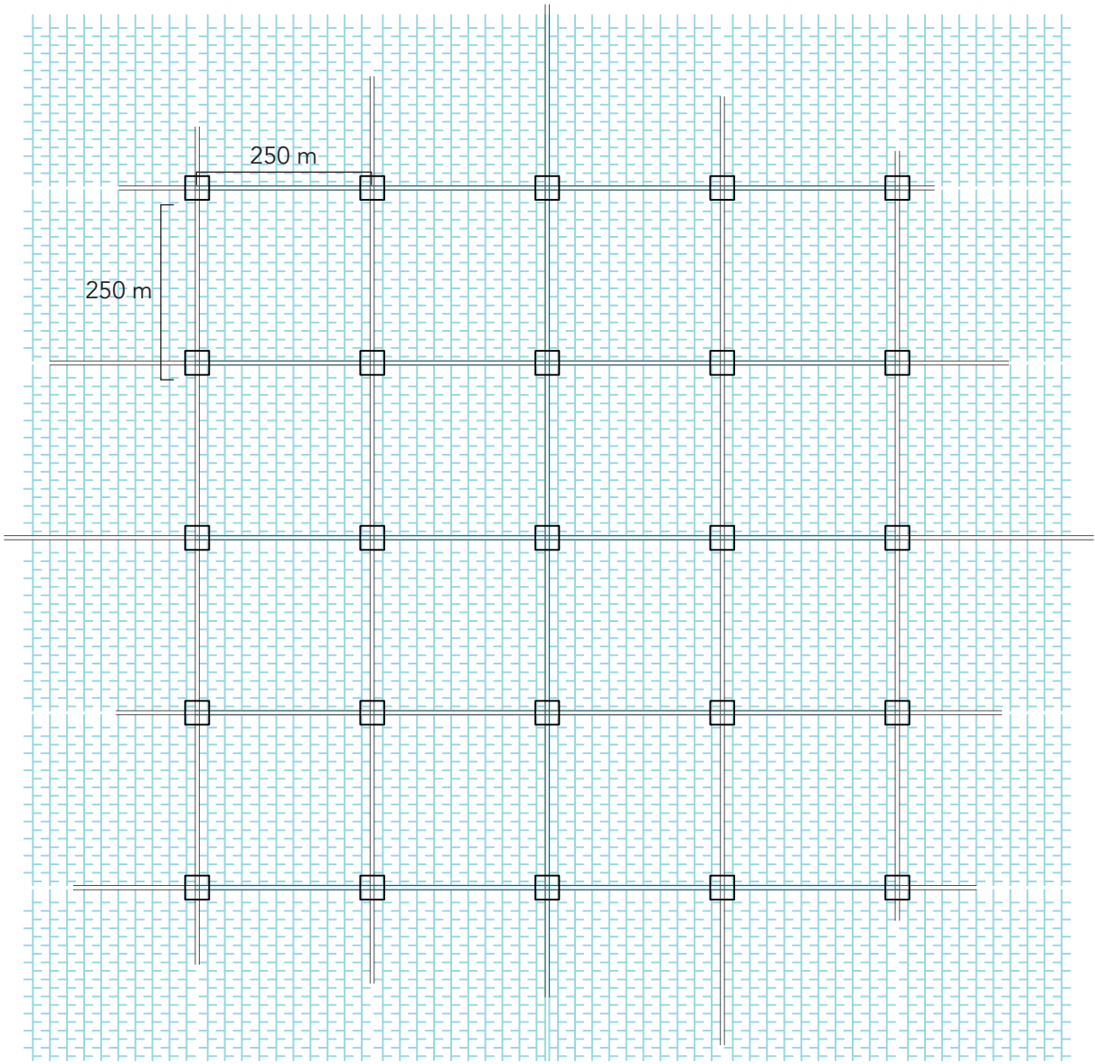
Réseau d'eau claire
