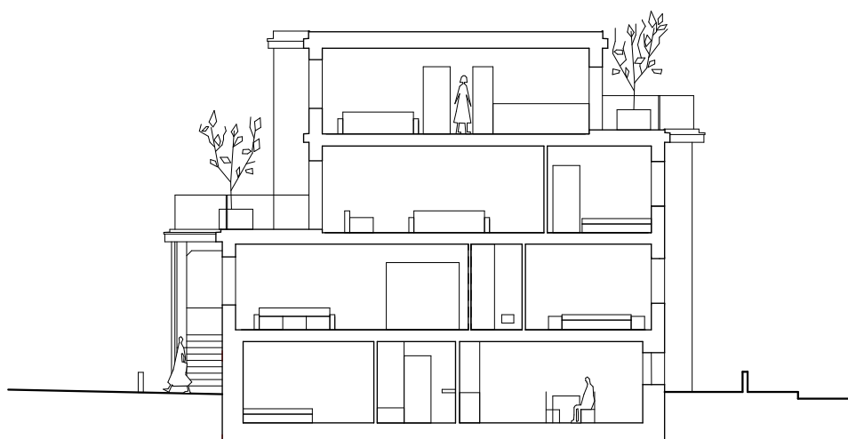
COUPE AA 1/200
