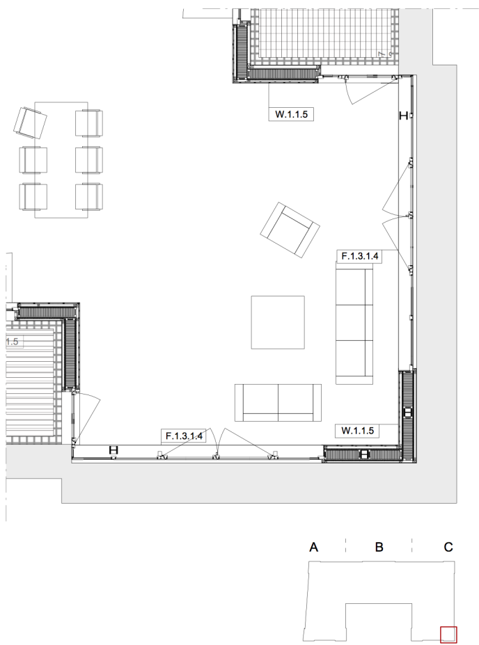
GRUNDRISSANSICHT "ECKRISALIT" Mst. 1:100
