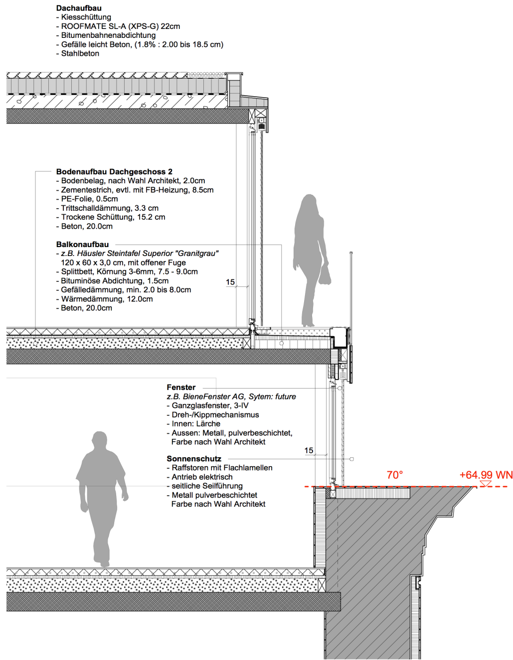
DETAILSCHNITT "ECKRISALIT" Mst. 1:50
