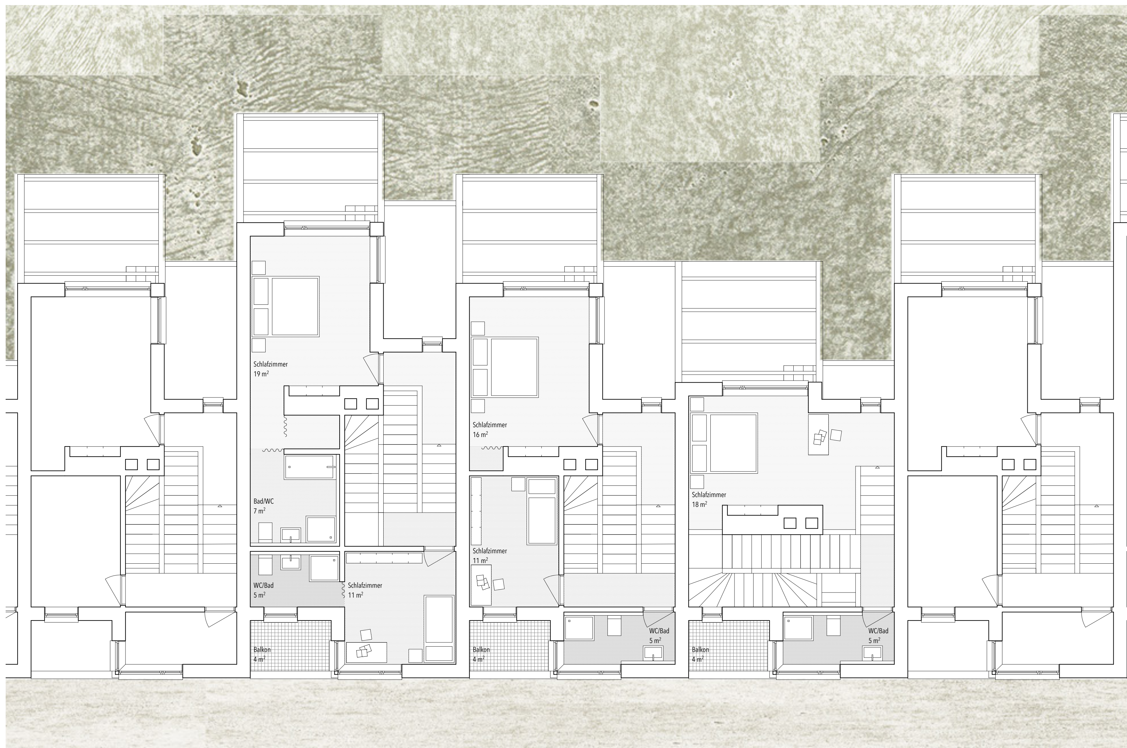
Raumtypologie 2. Obergeschoss 1:66
