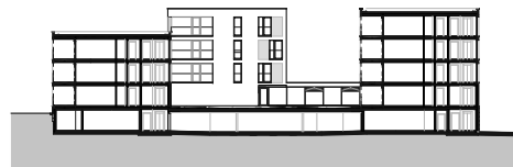
Schnitt 2
