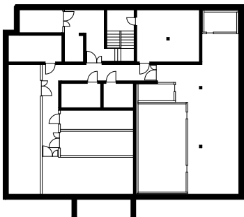
Untergeschoss
