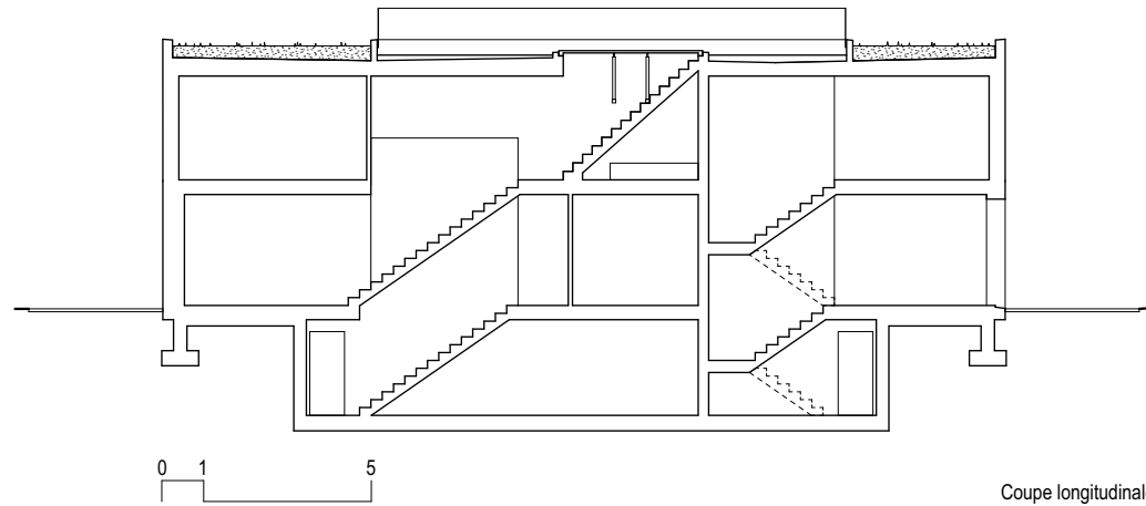
Coupe longitudinale
