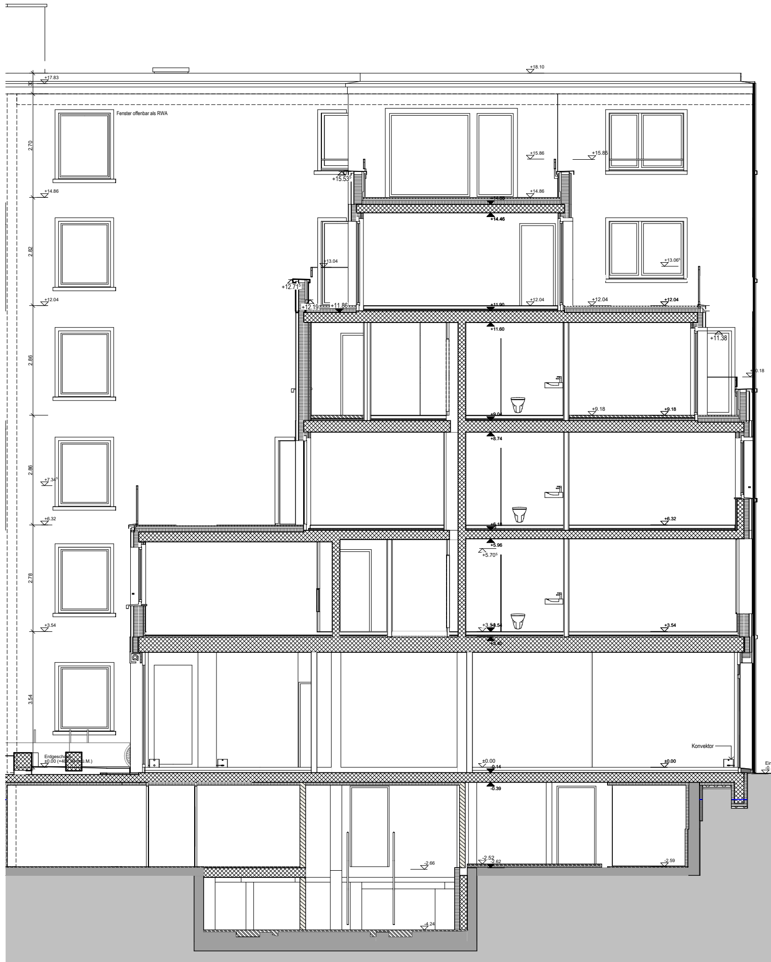
Schnitt-Ansicht detailliert
