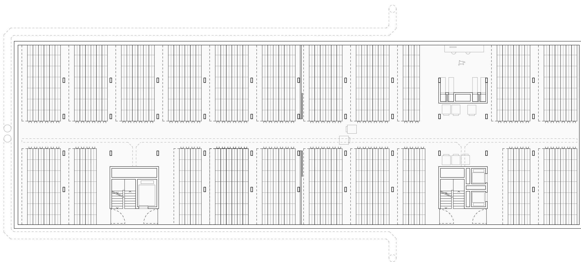
sous-sol type locaux de stockage livres
