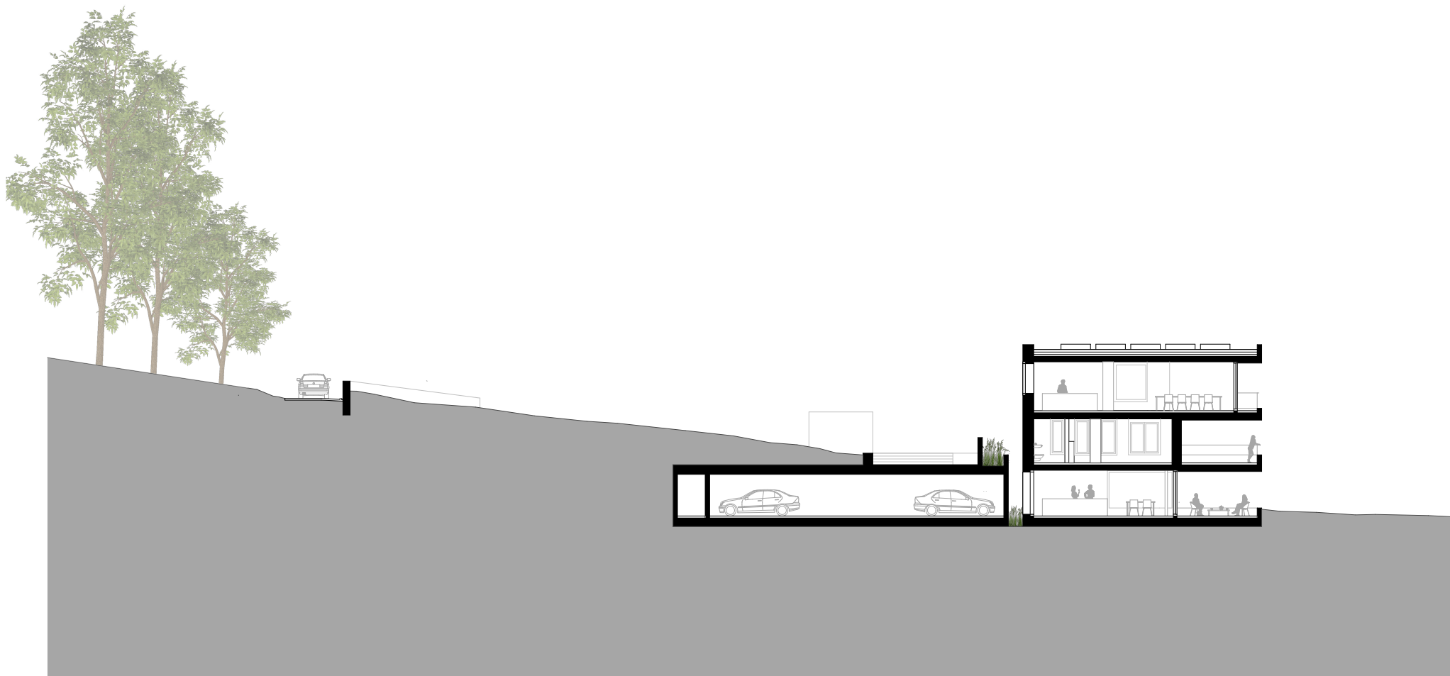
Längsschnitt
