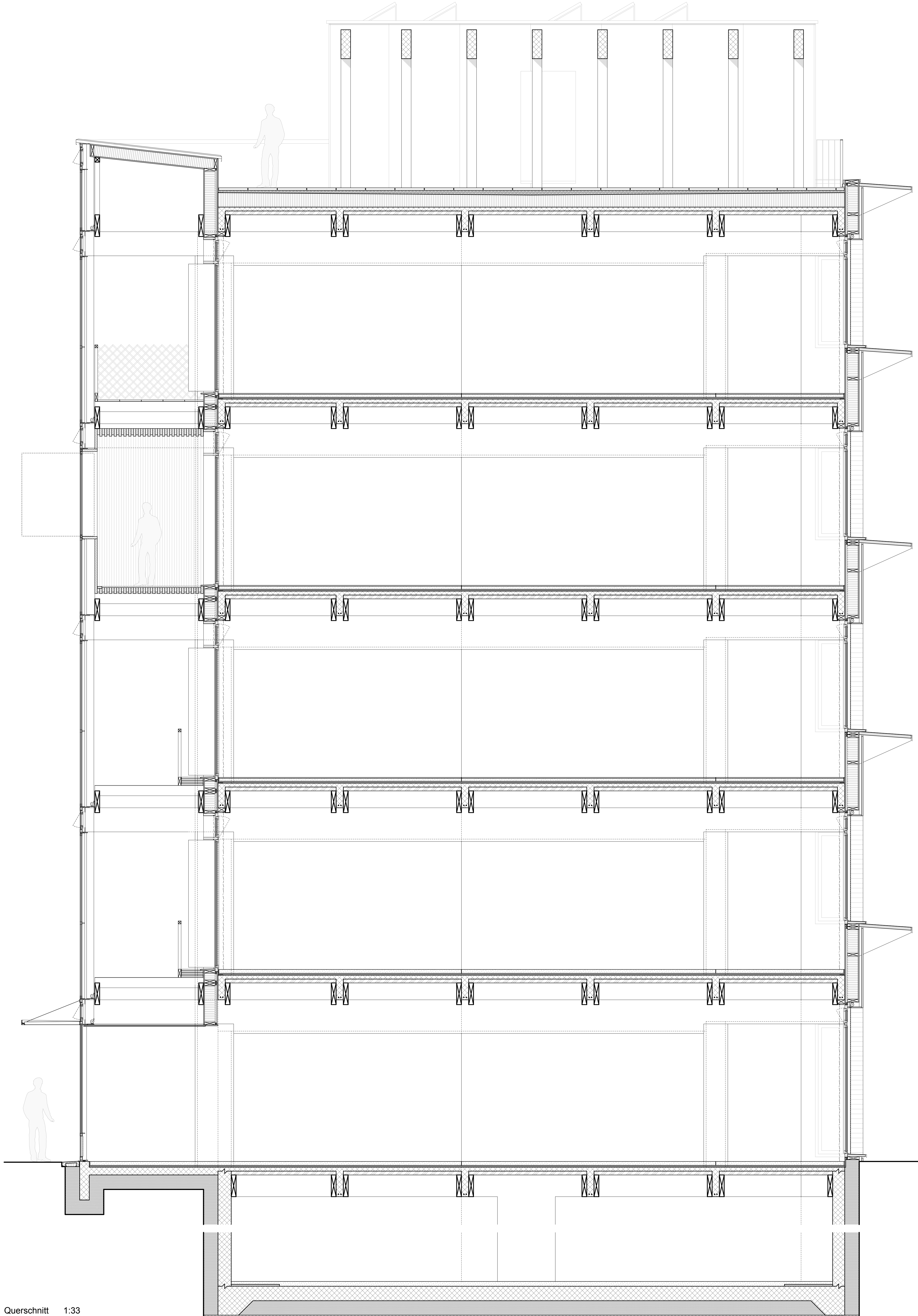
Querschnitt 1:33
