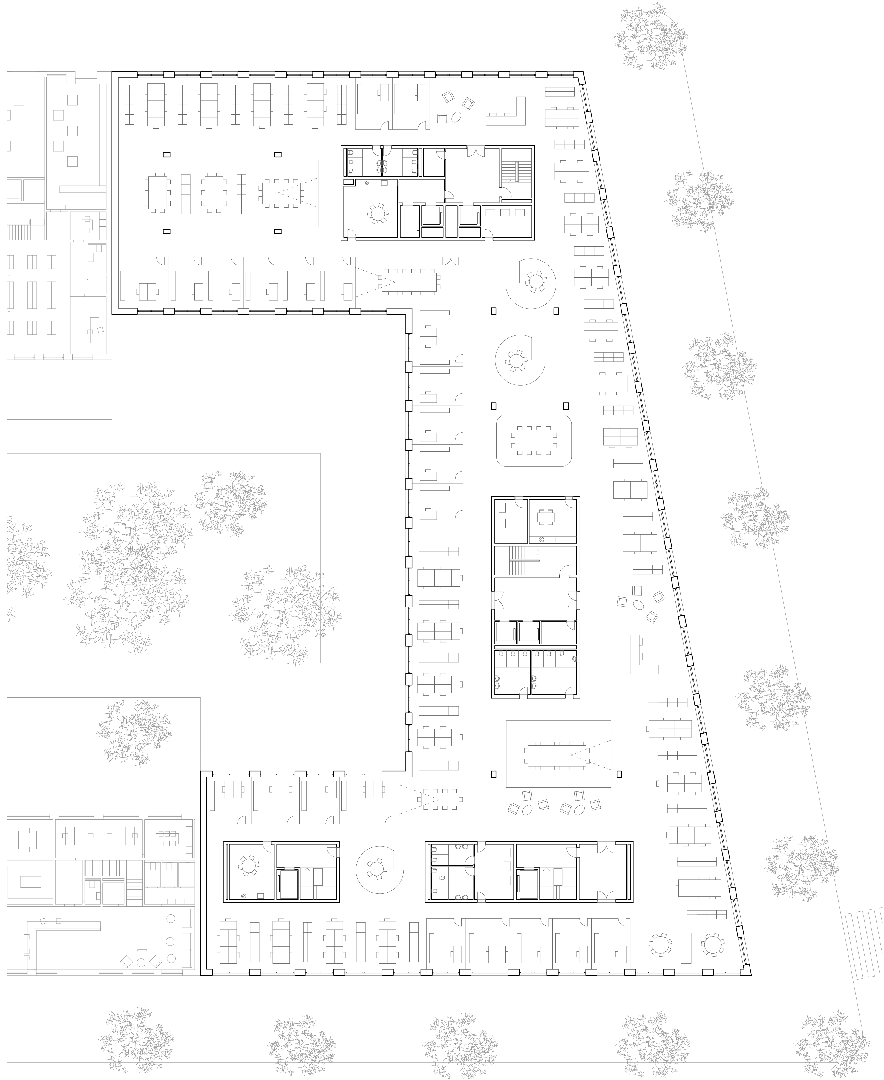
NIVEAU 1 1:200
