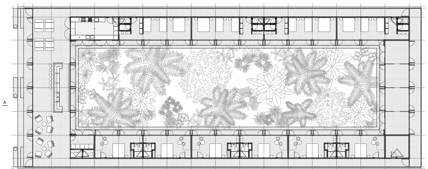
Erdgeschoss | Rez-de-chaussée
