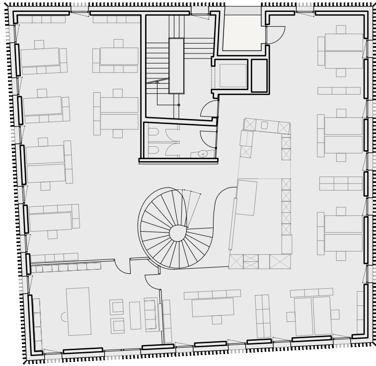
1. Obergeschoss [Büro] 1:200
