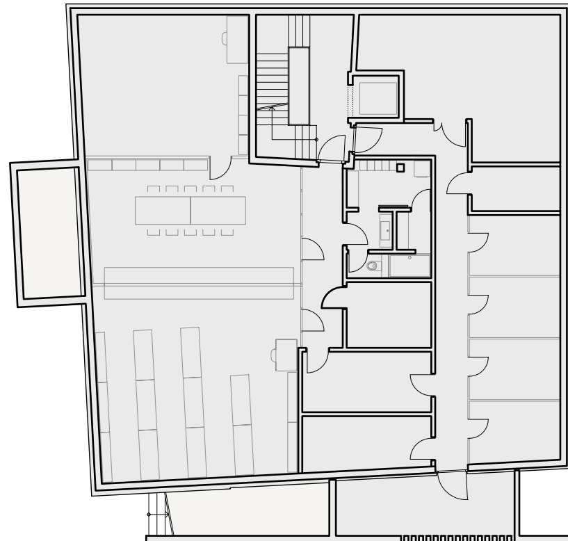
1. Untergeschoss 1:200
