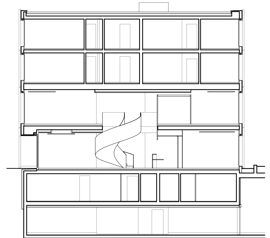
Schnitt 1:200
