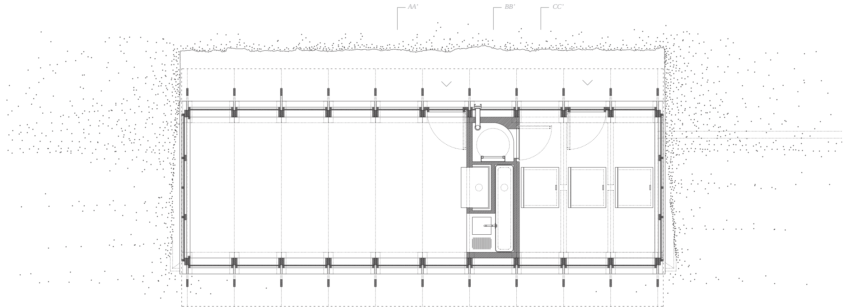
Plan niveau \pm 0.00 - échelle 1.50 -
