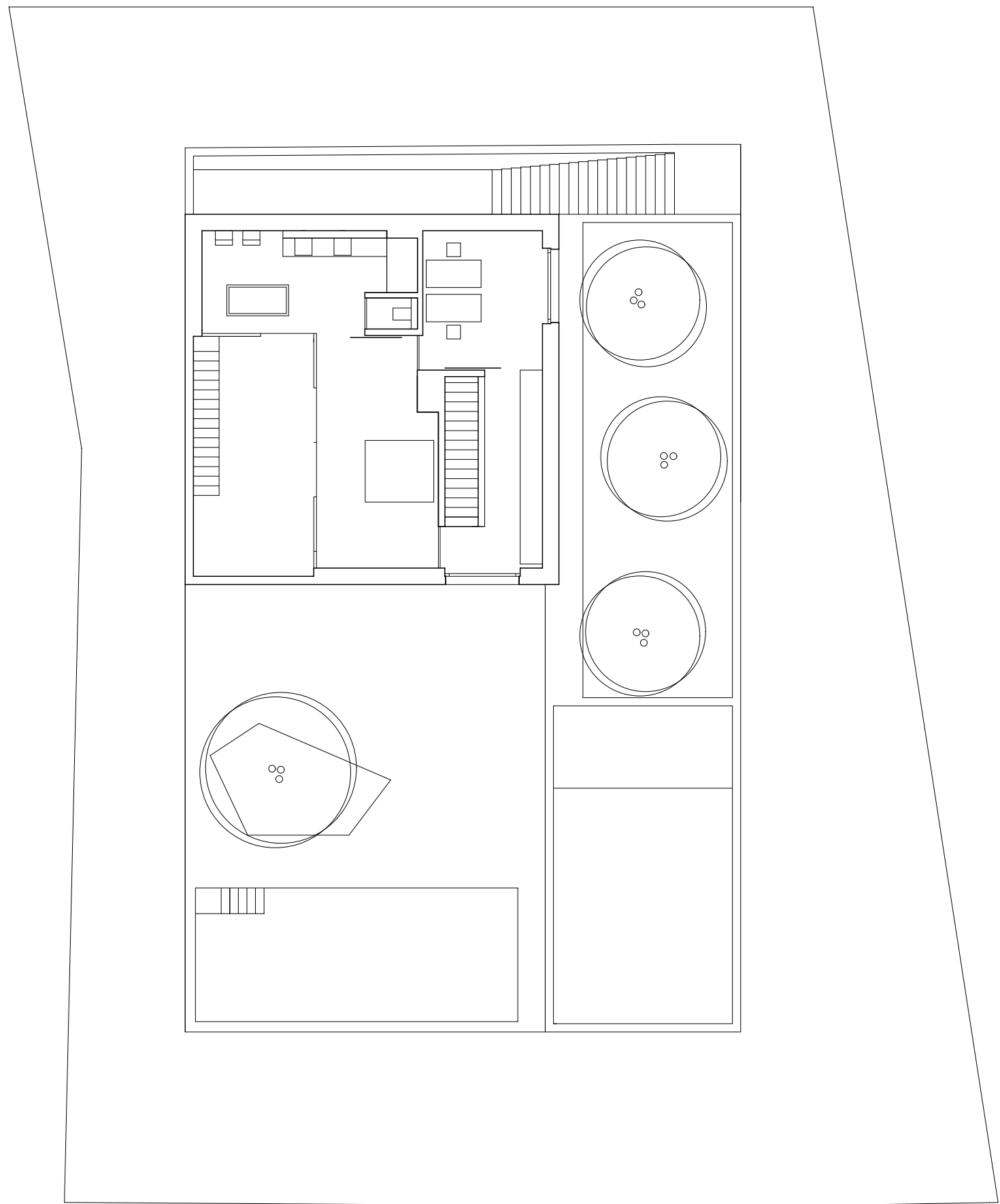
OBERGESCHOSS 1:150
