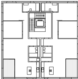
Grundrisse Haus B3 M 1:100
