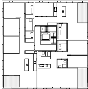
Grundrisse Haus A3 M 1:100
