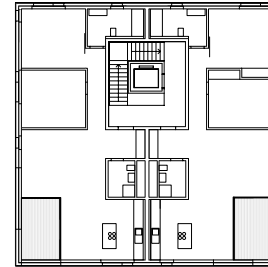
Grundrisse Haus B2 M 1:100
