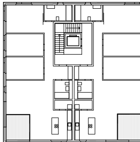
Grundrisse Haus C1 M 1:100
