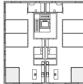
Grundrisse Haus C2 M 1:100
