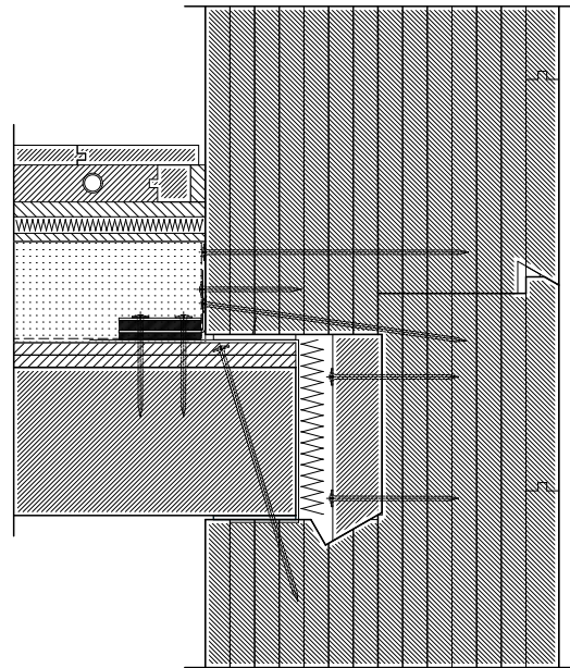
Geschossübergang
