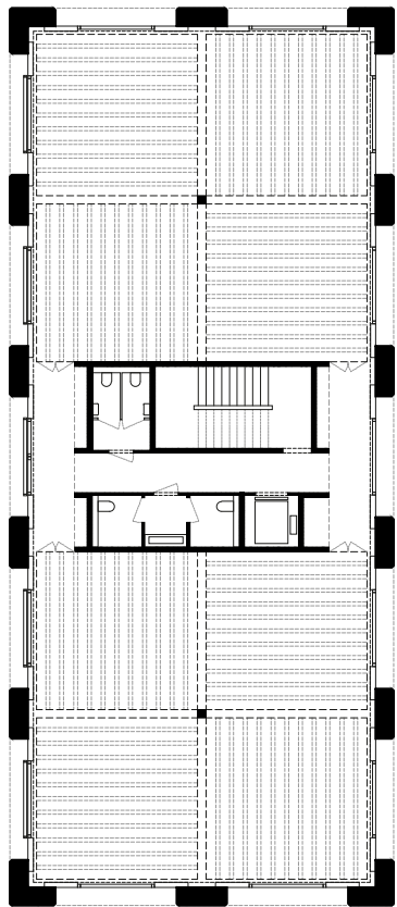
2. Obergeschoss | 2 ème étage
