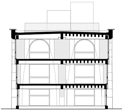
Schnitt A | Coupe A
