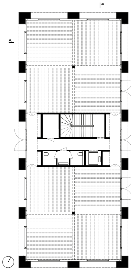
Erdgeschoss | Rez-de-chaussée
