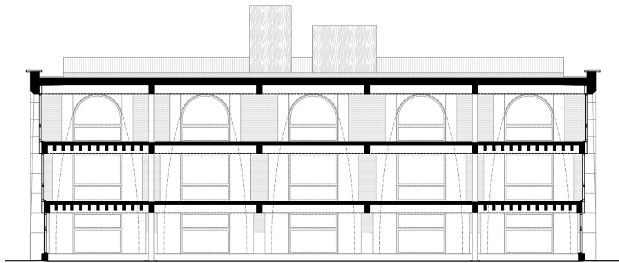
Schnitt B | Coupe B
