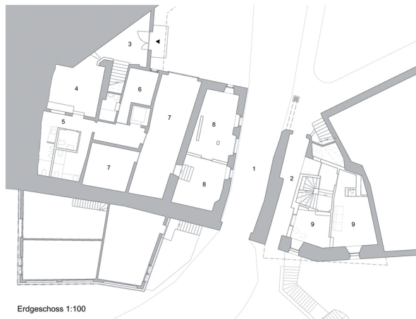
Erdgeschoss 1:100
