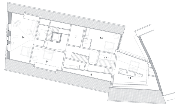
Dachgeschoss 1:100
