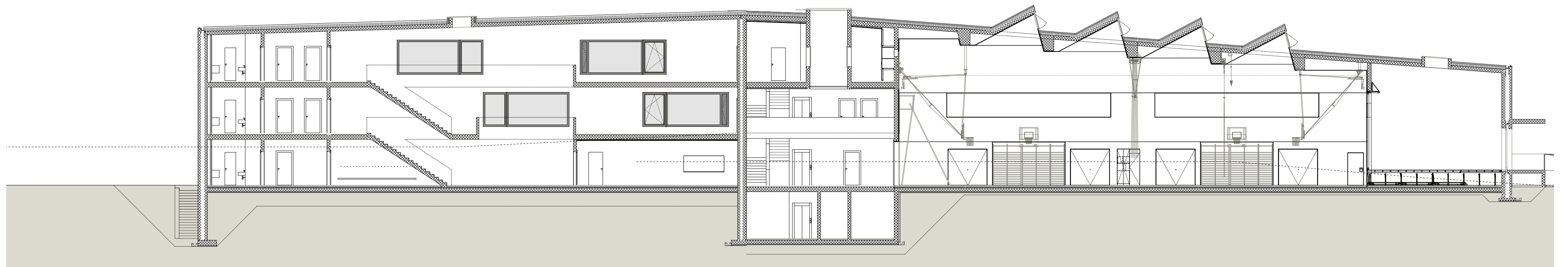
COUPE LONGITUDINALE
