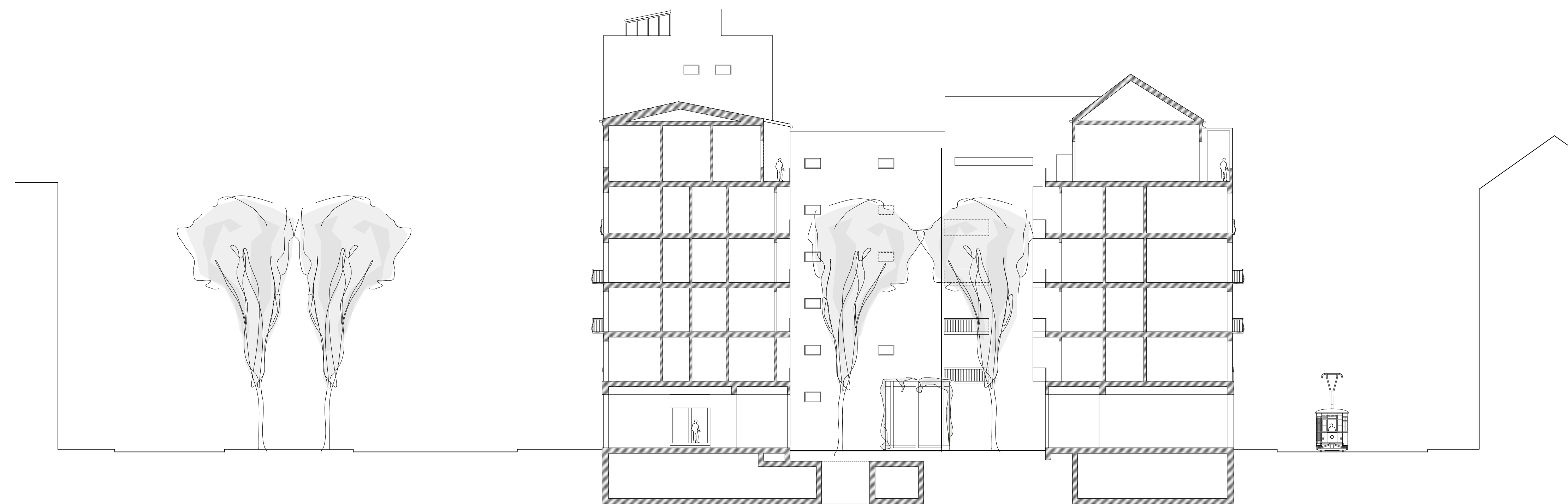
Querschnitt 1 : 200
