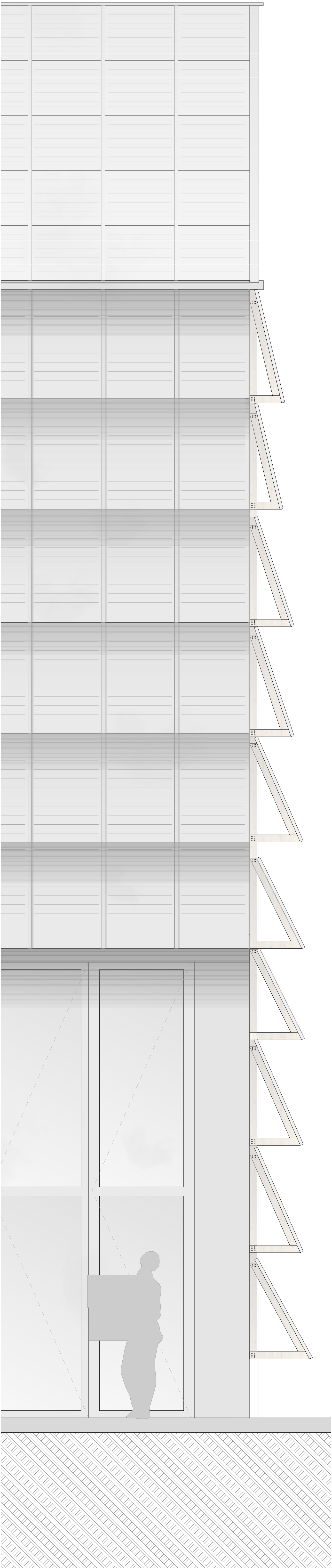
Façade Sud - 1:20
