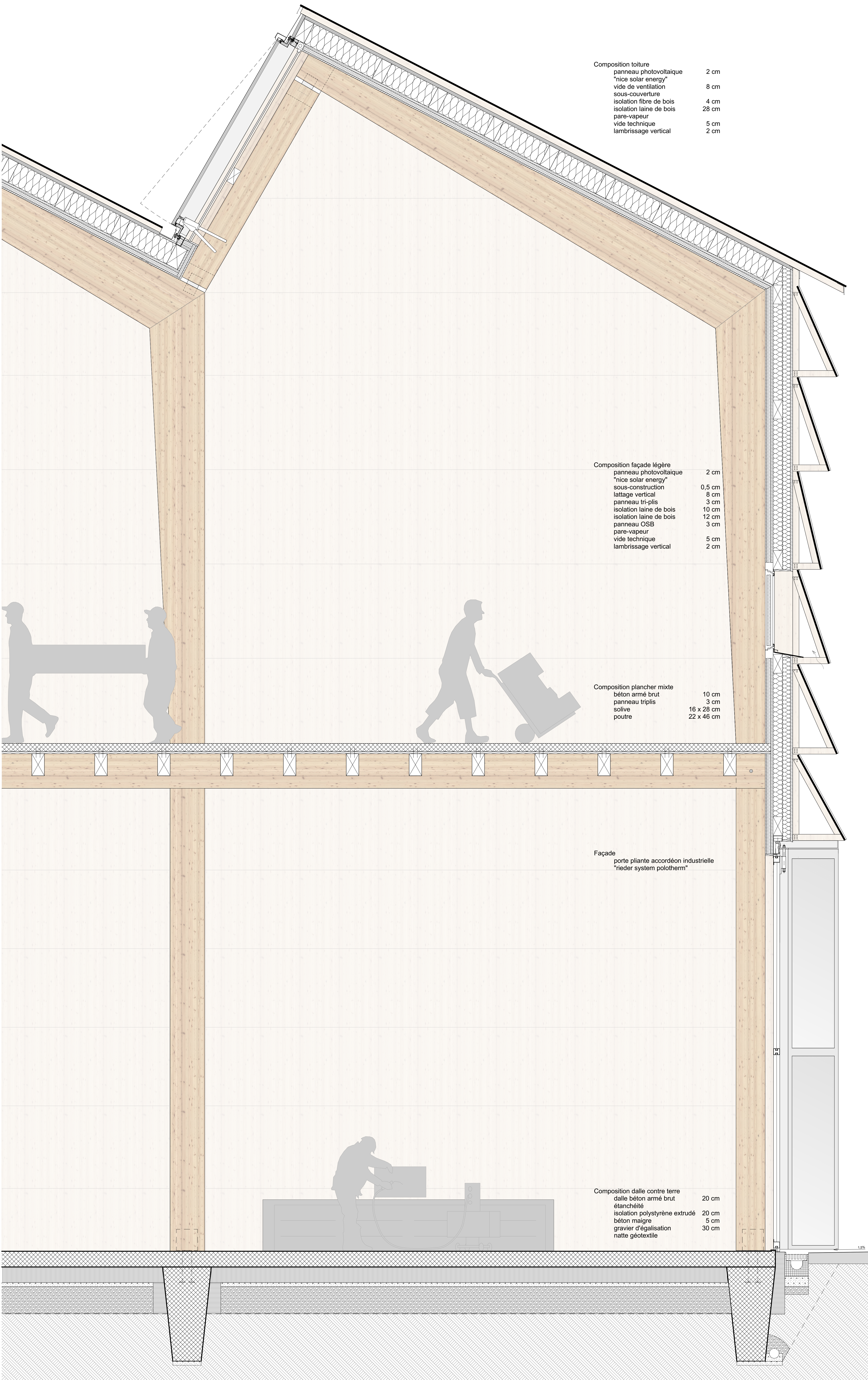
Travée Sud - 1:20
