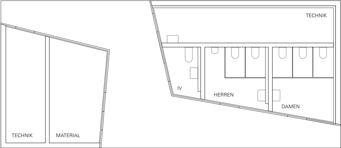
GRUNDRISS
