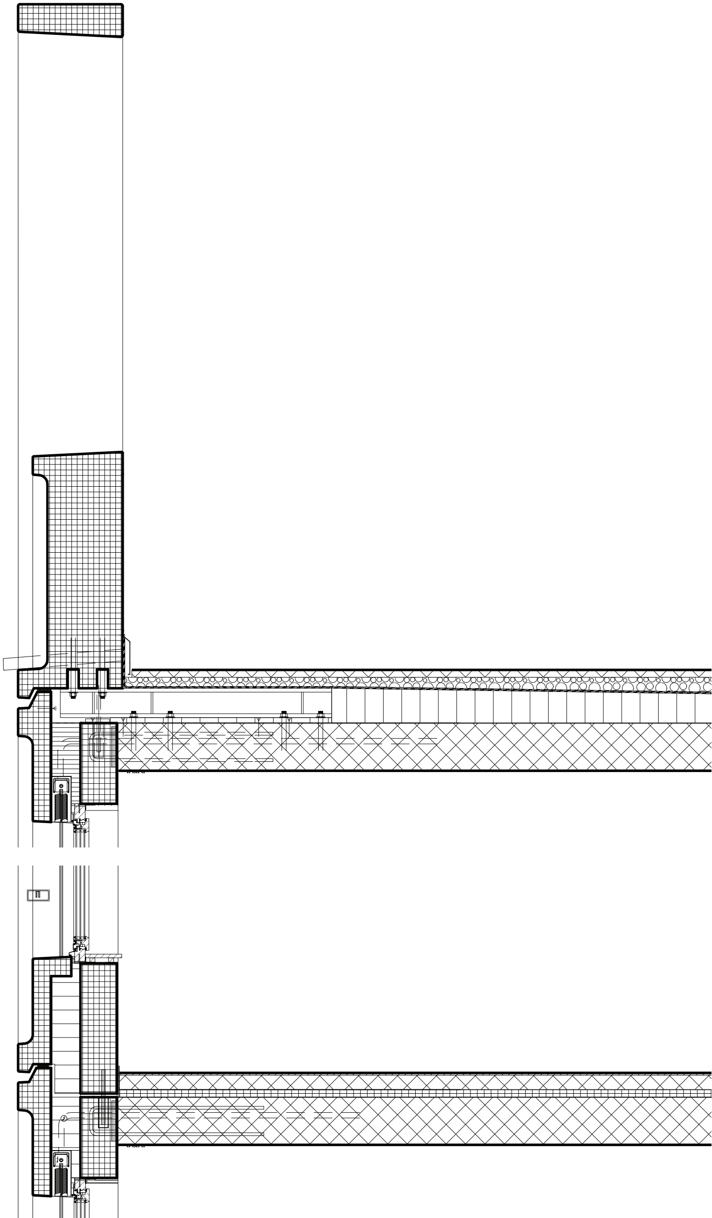
Schnitt 1:20
