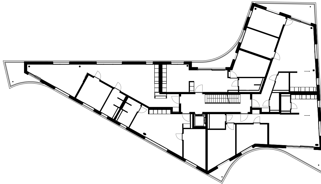
Grundriss 1.OG - 3.OG M 1:400
