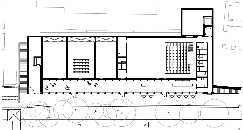
Erdgeschoss | Rez-de-chaussée
