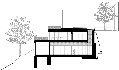
Schnitt A | Coupe A
