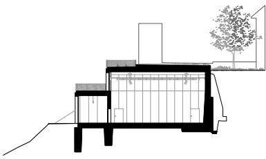
Schnitt B | Coupe B
