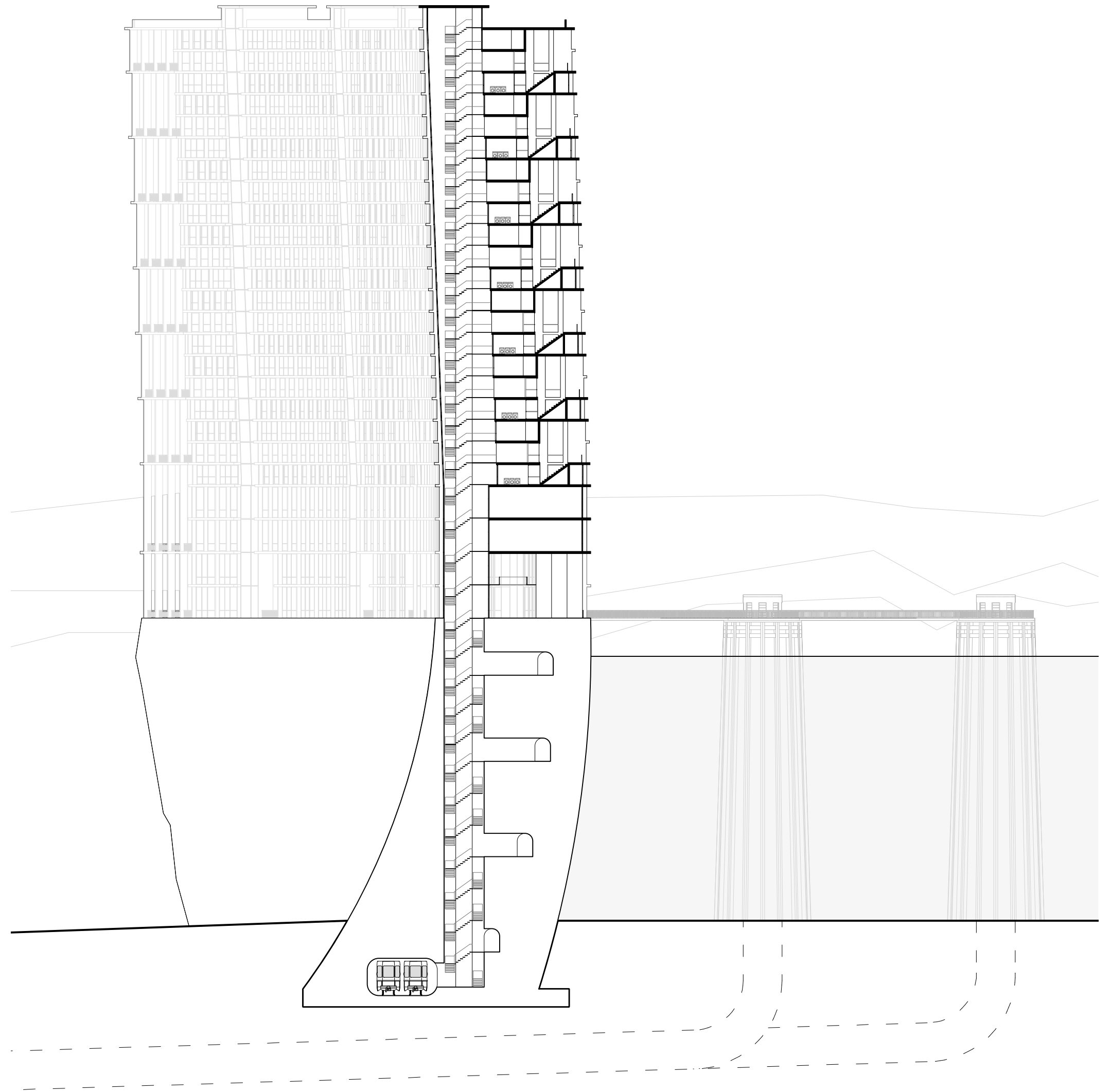
Schnitt B-B 1:500
