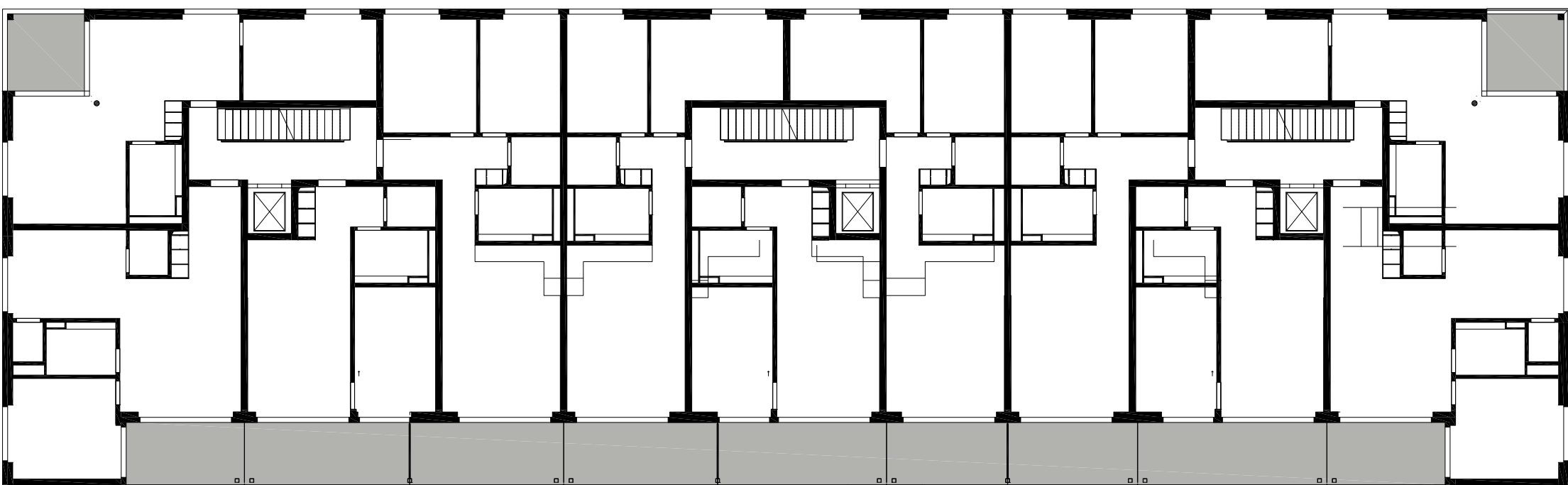
Regelgeschoss
