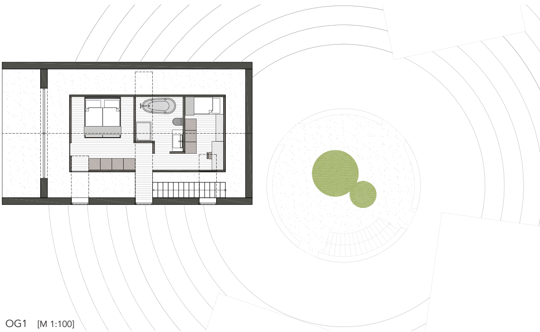
OG1 [M 1:100]
