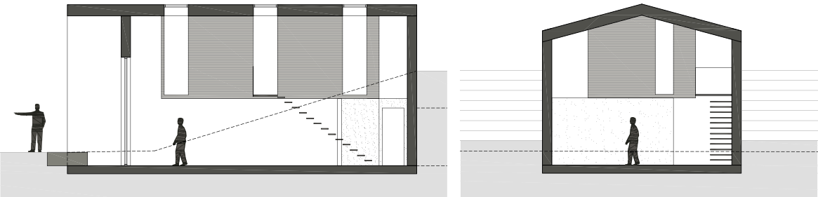
SCHNITT 1-1 [M 1:100]
