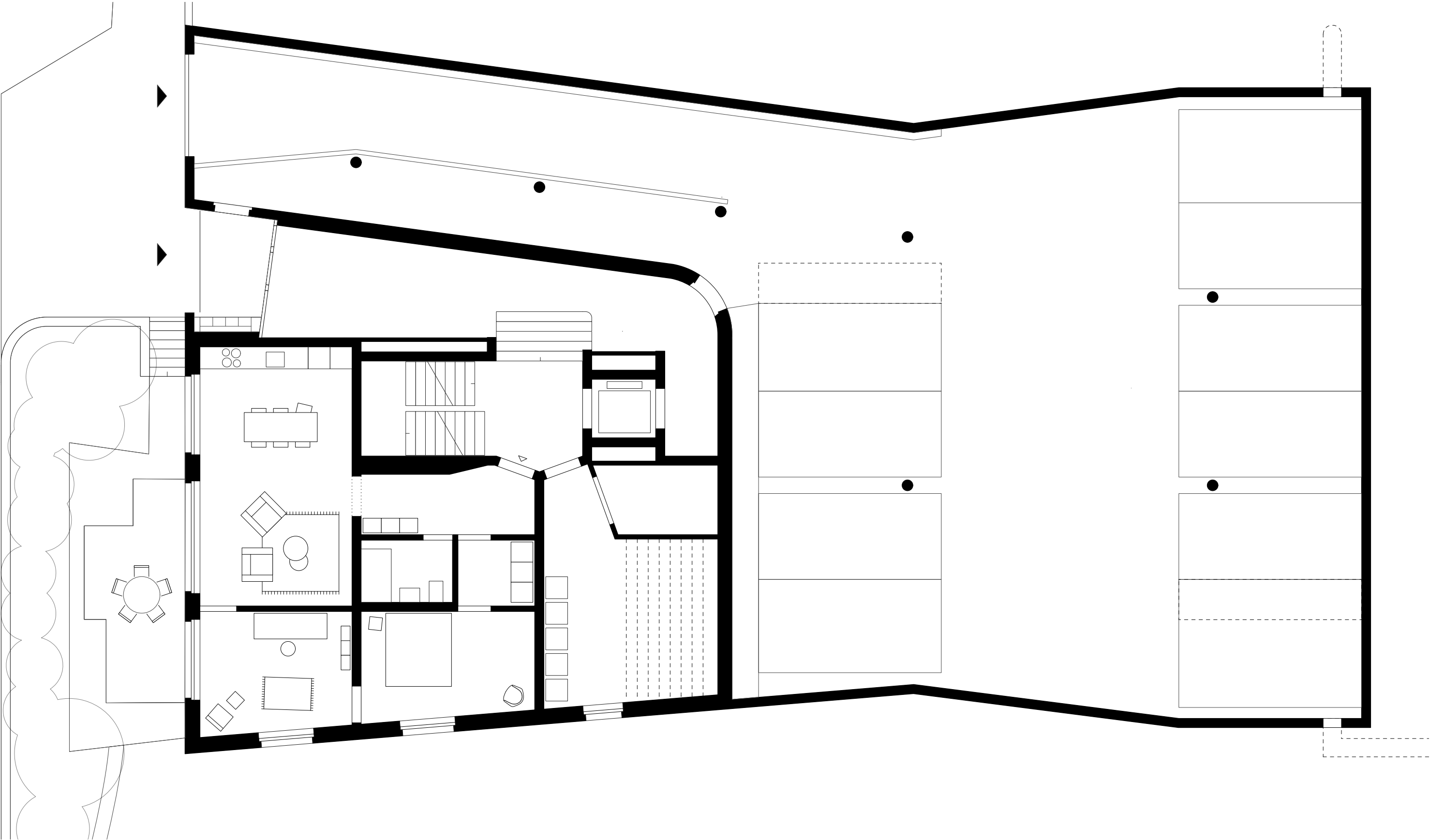
1. UNTERGESCHOSS, 1:100
