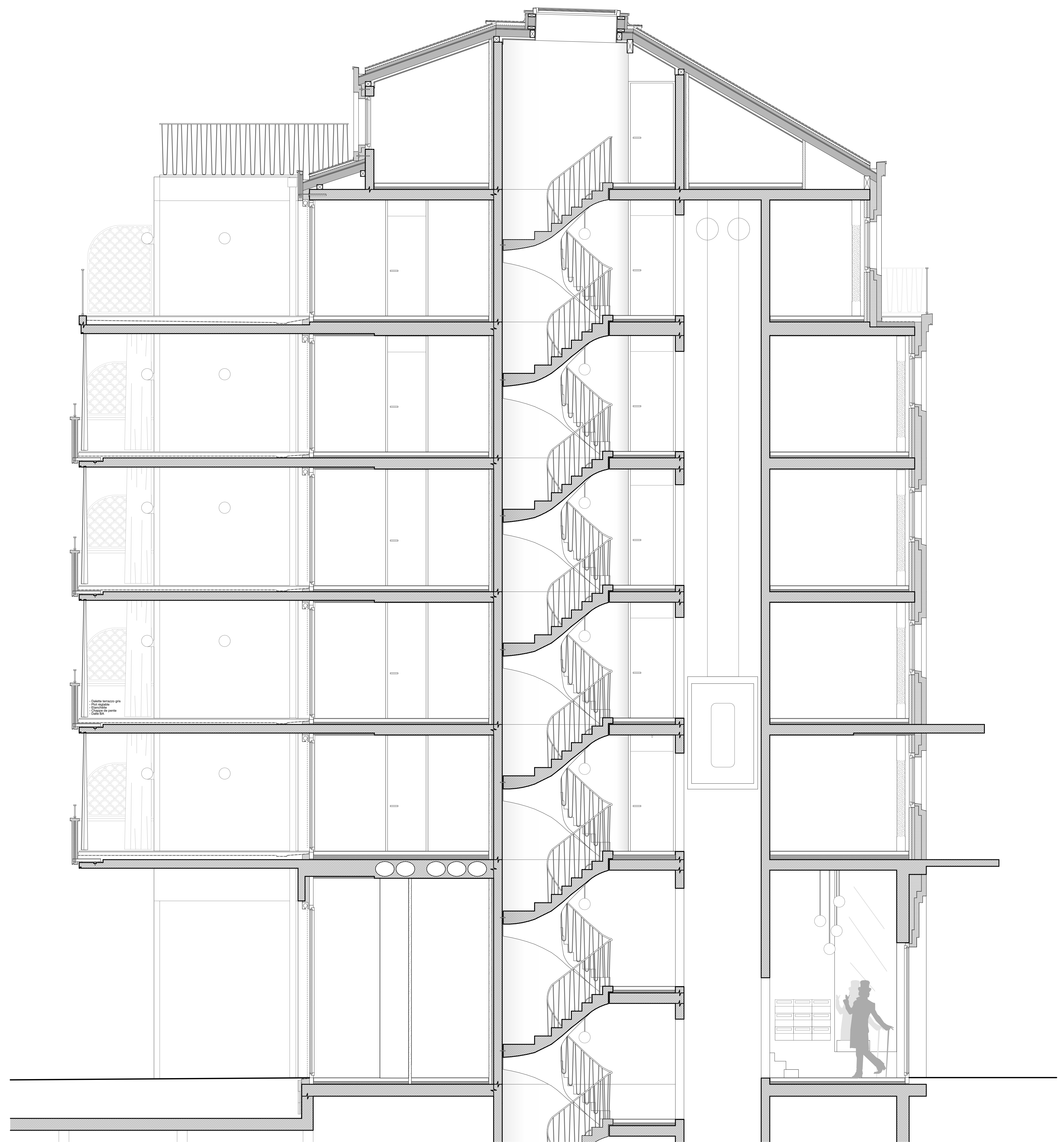
Façade et coupe constructive sur cour
