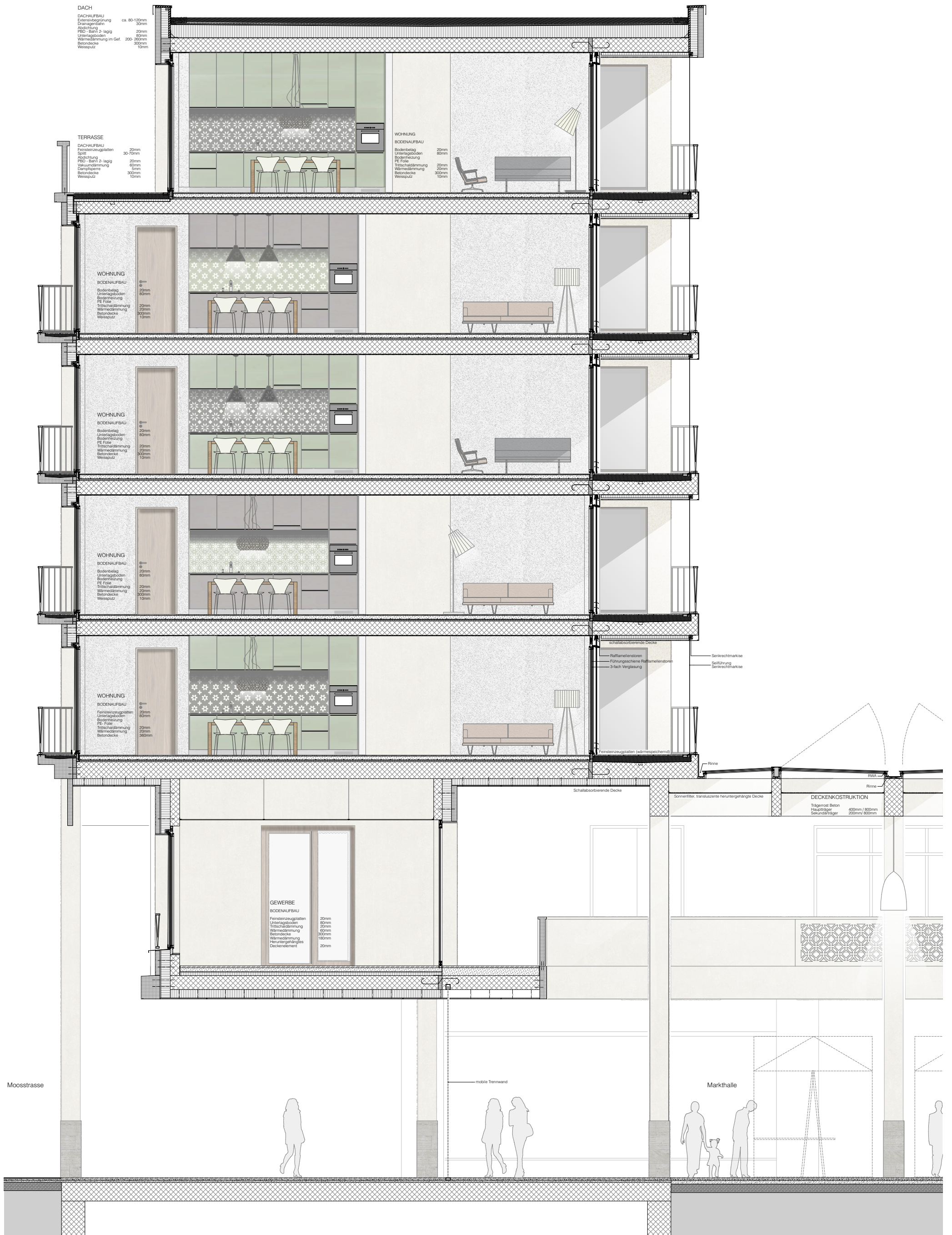
Konstruktionsschnitt
