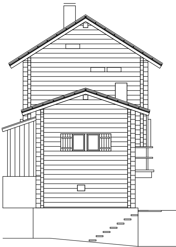
façade Ouest
