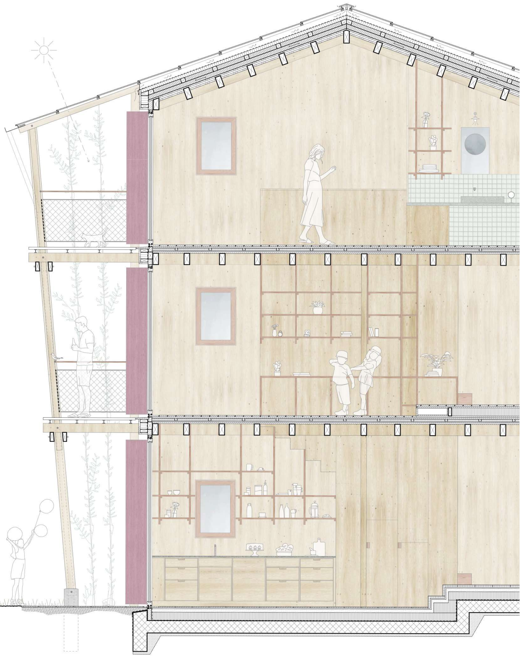
Fassaderschnitt 1:33
