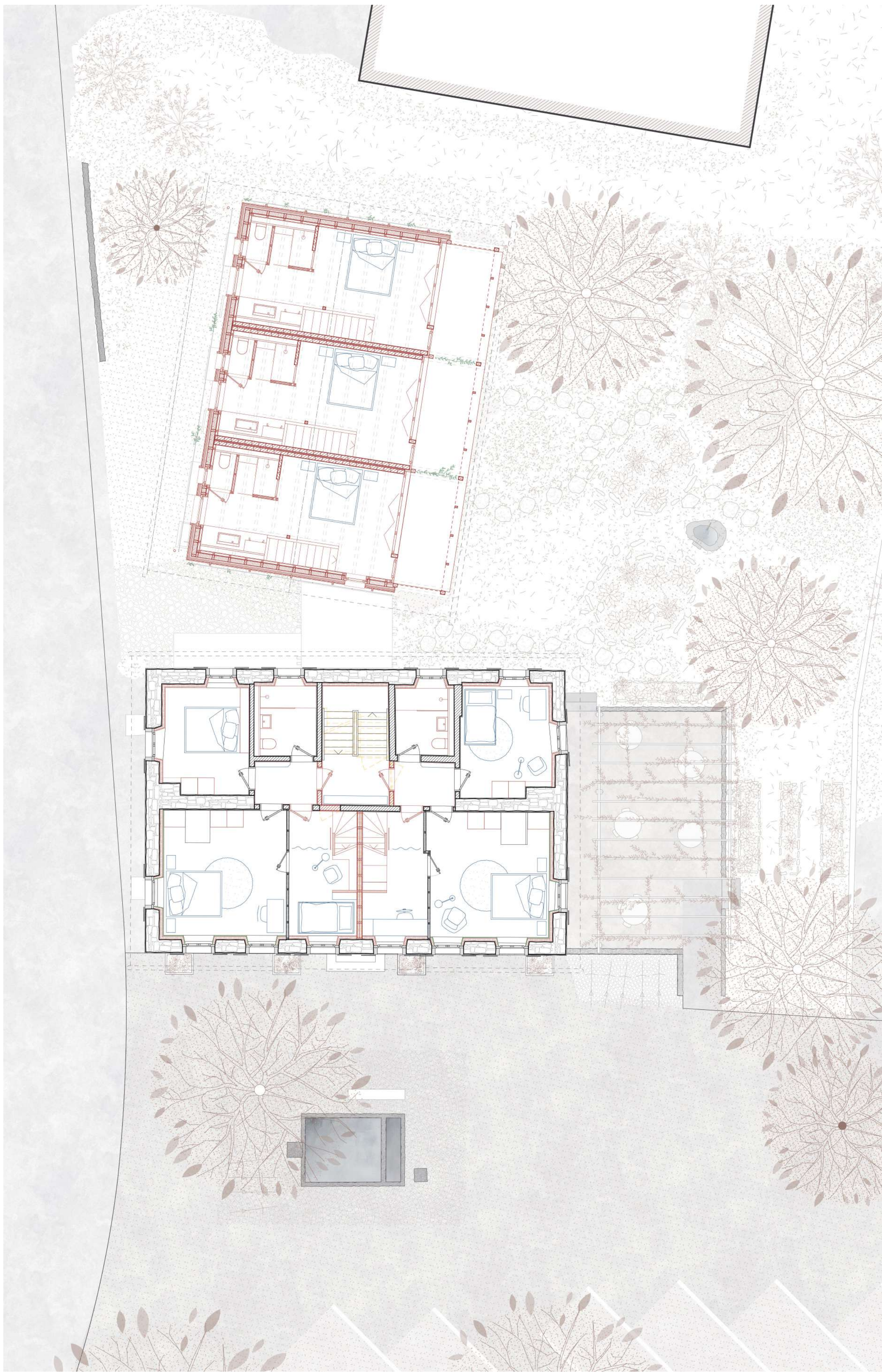
Grundriss 2. Obergeschoss 1:100
