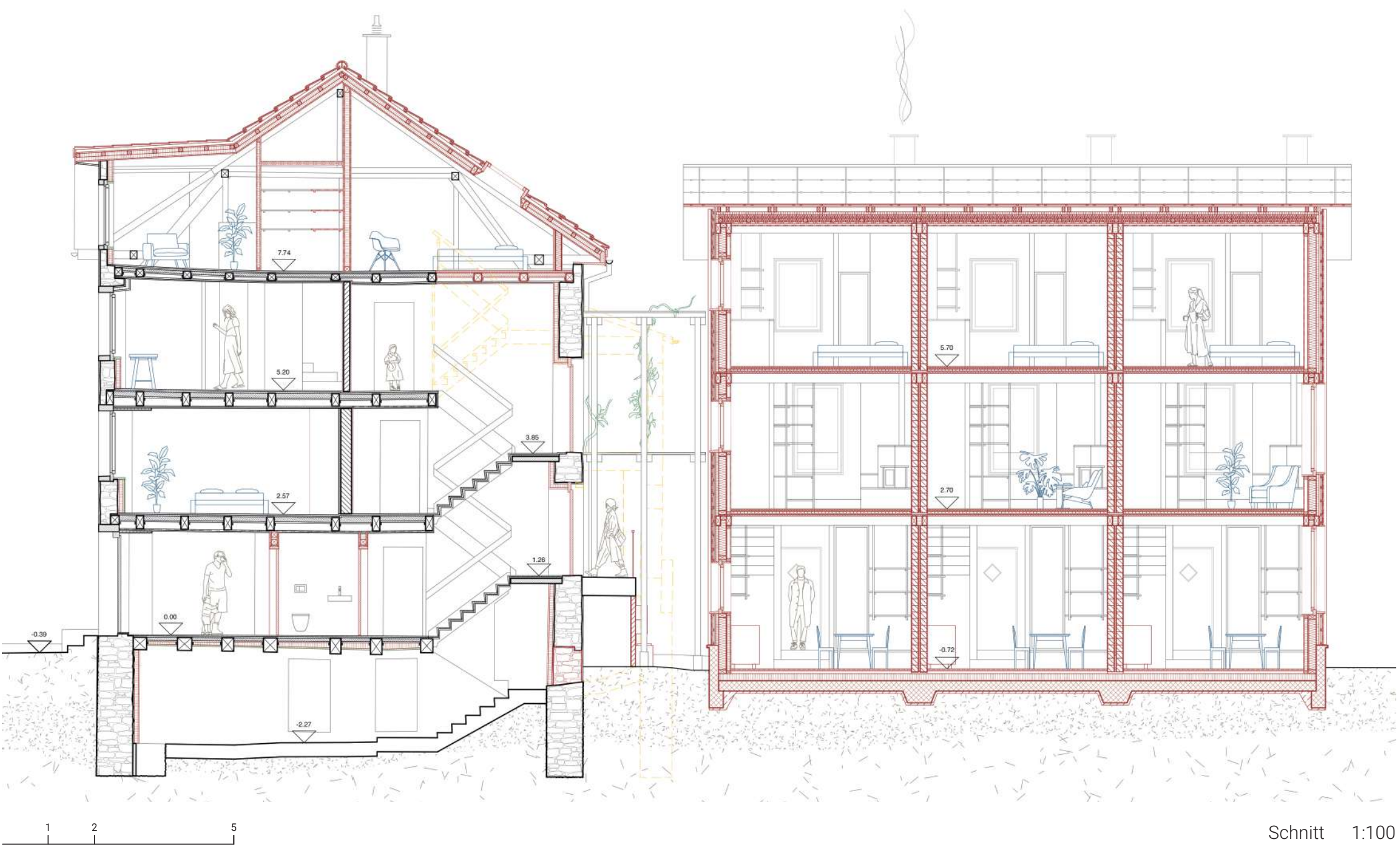
Schnitt 1:100
