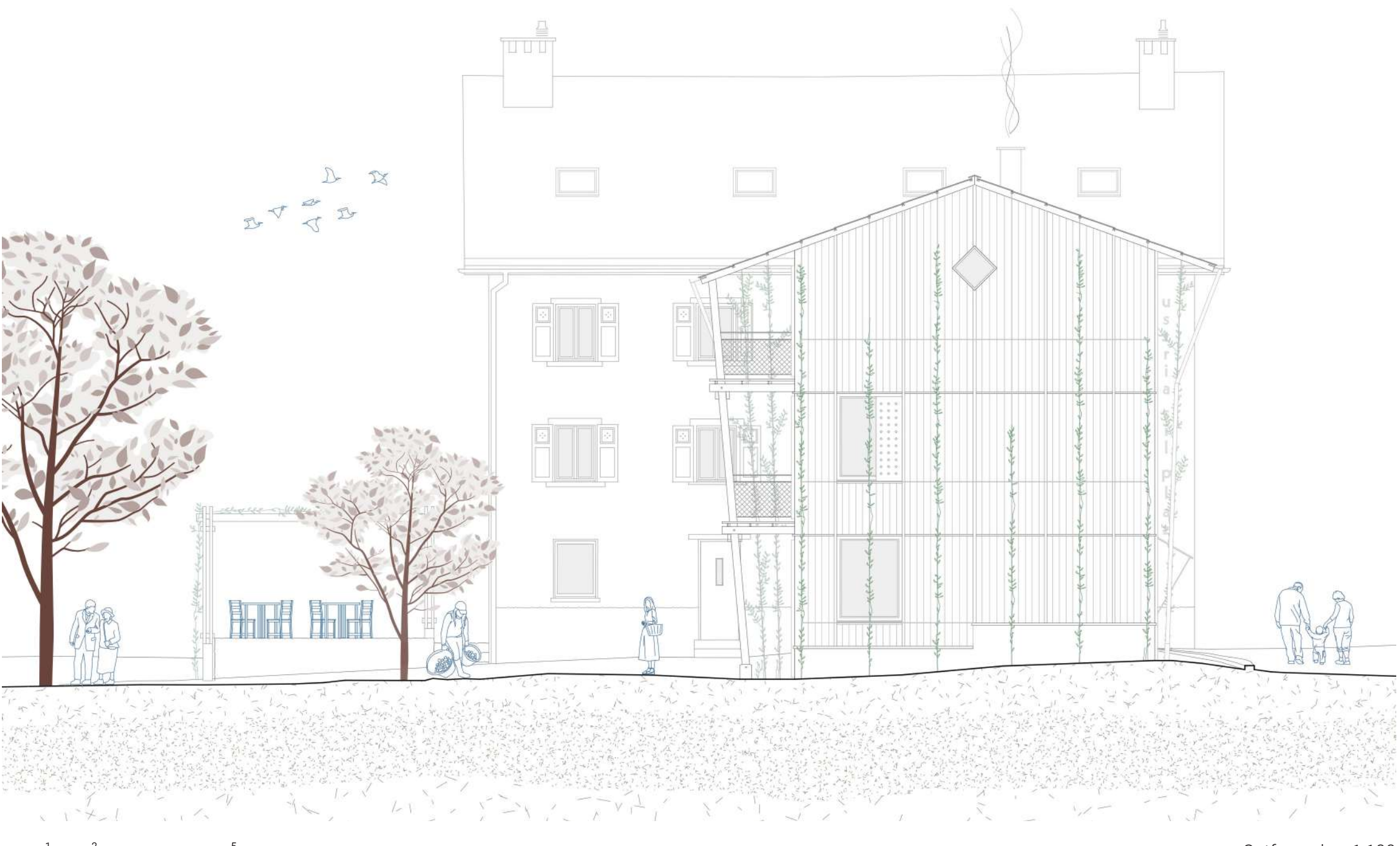
Ostfassade 1:100
