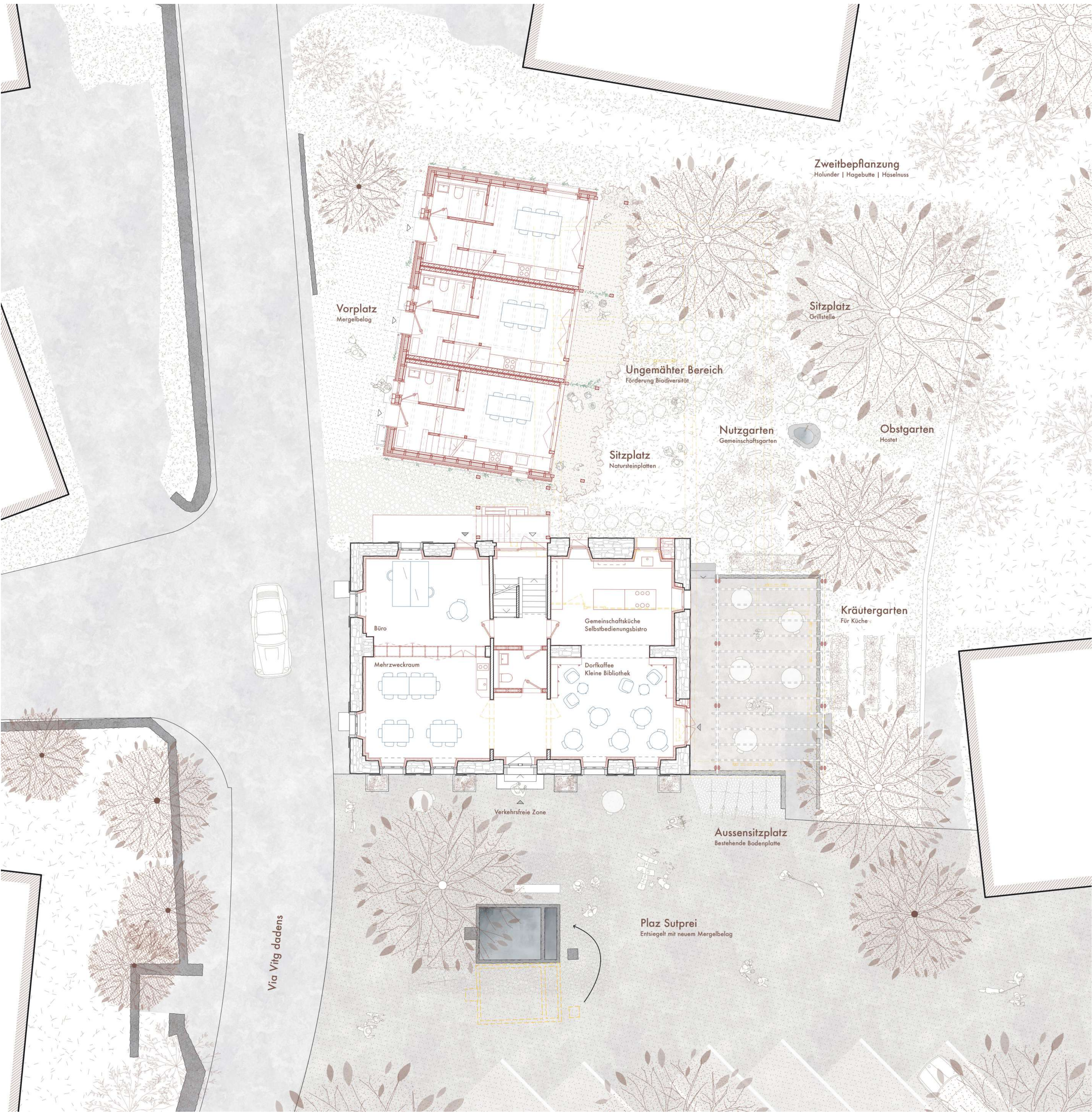
Grundriss Erdgeschoss mit Umgebung 1:100
