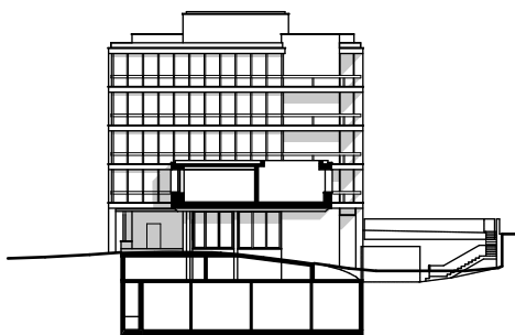
Südwestansicht I M1:700
