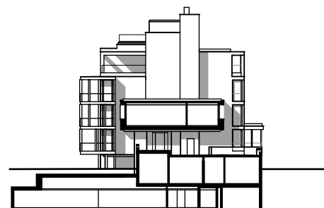
Nordostansicht II M1:700
