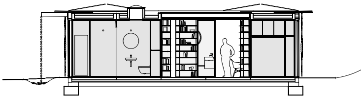
Längsschnitt Coupe longitudinale
