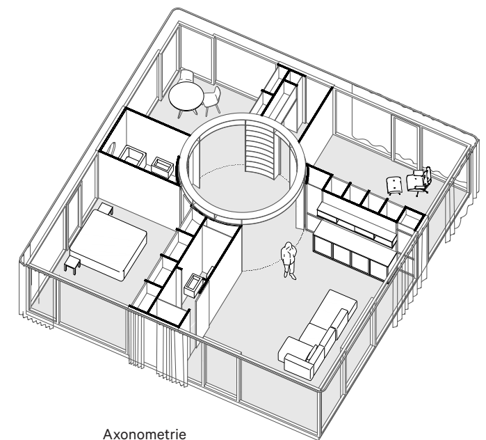
Axonometrie axonométrie
