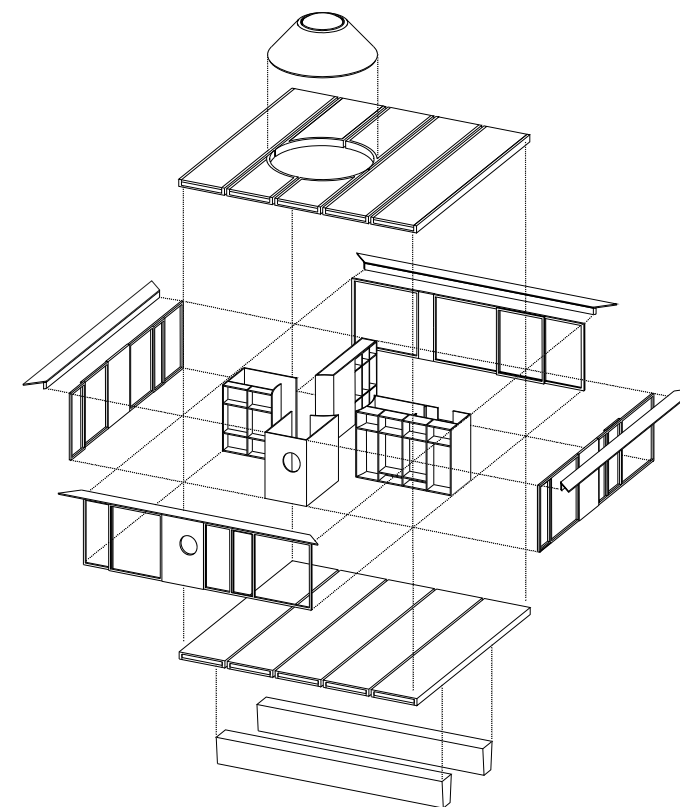
Bewegliche Elemente éléments mobiles
