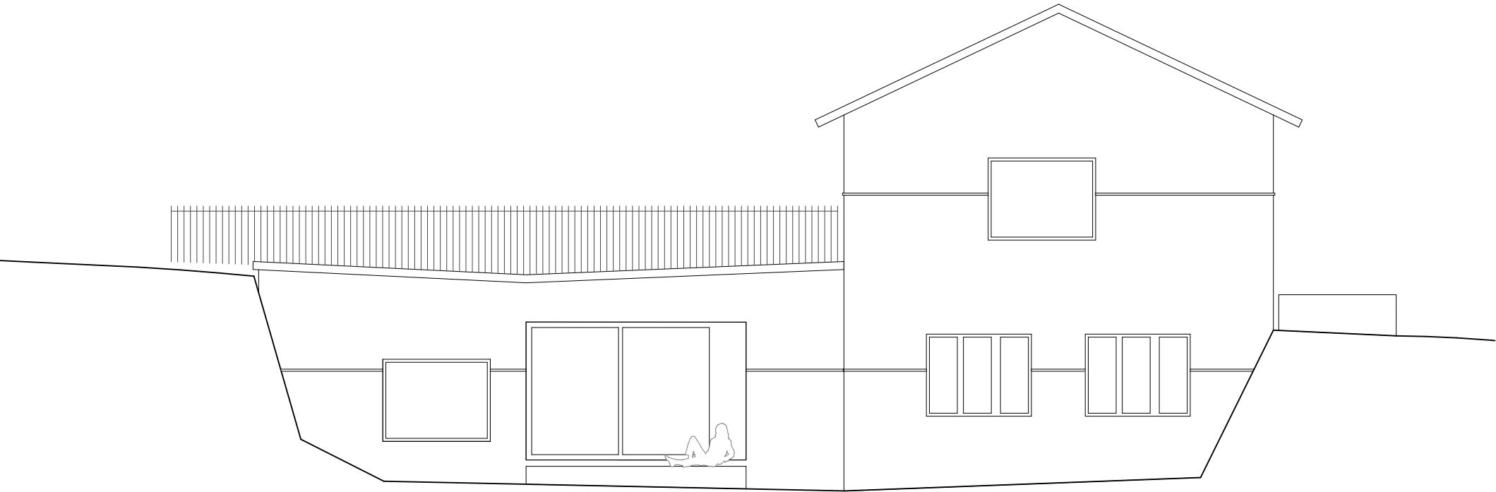
ELEVATION NORD-EST
