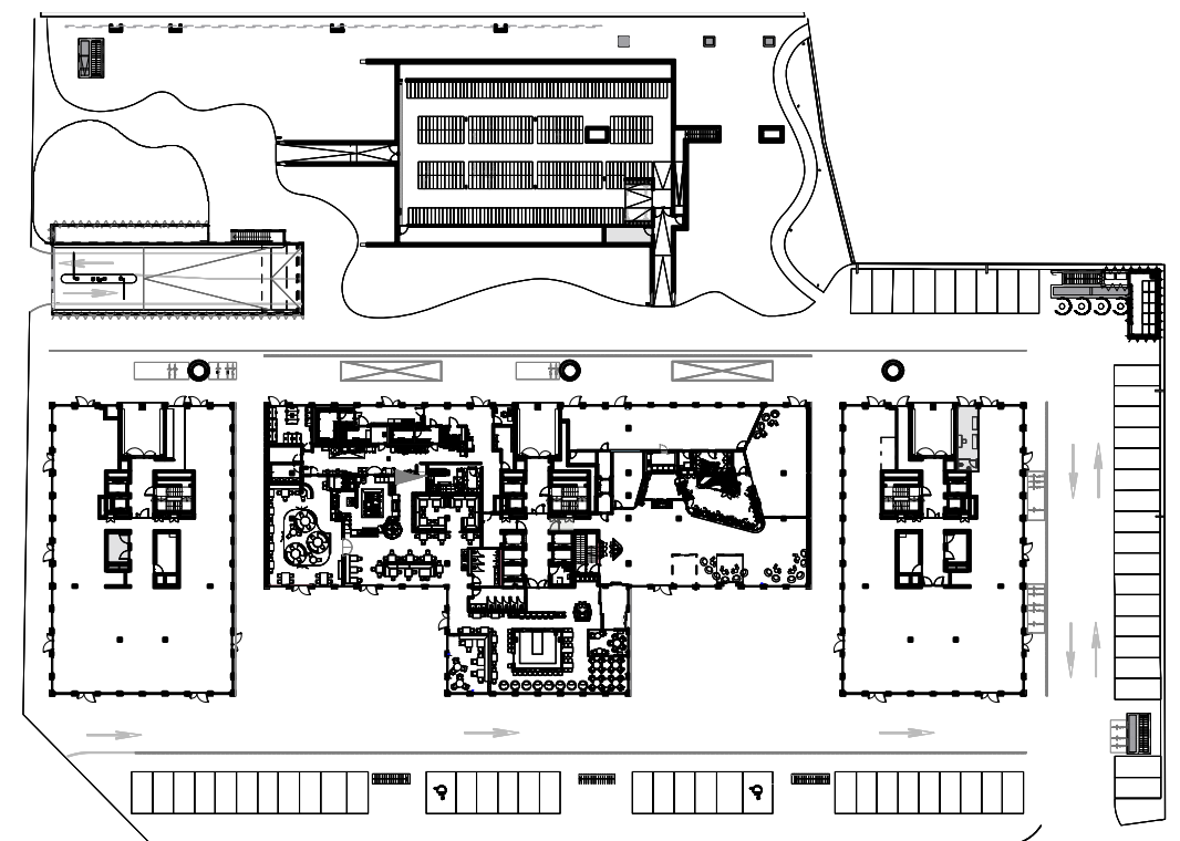
Übersicht Grundriss, Erdgeschoss MST. 1:1000
