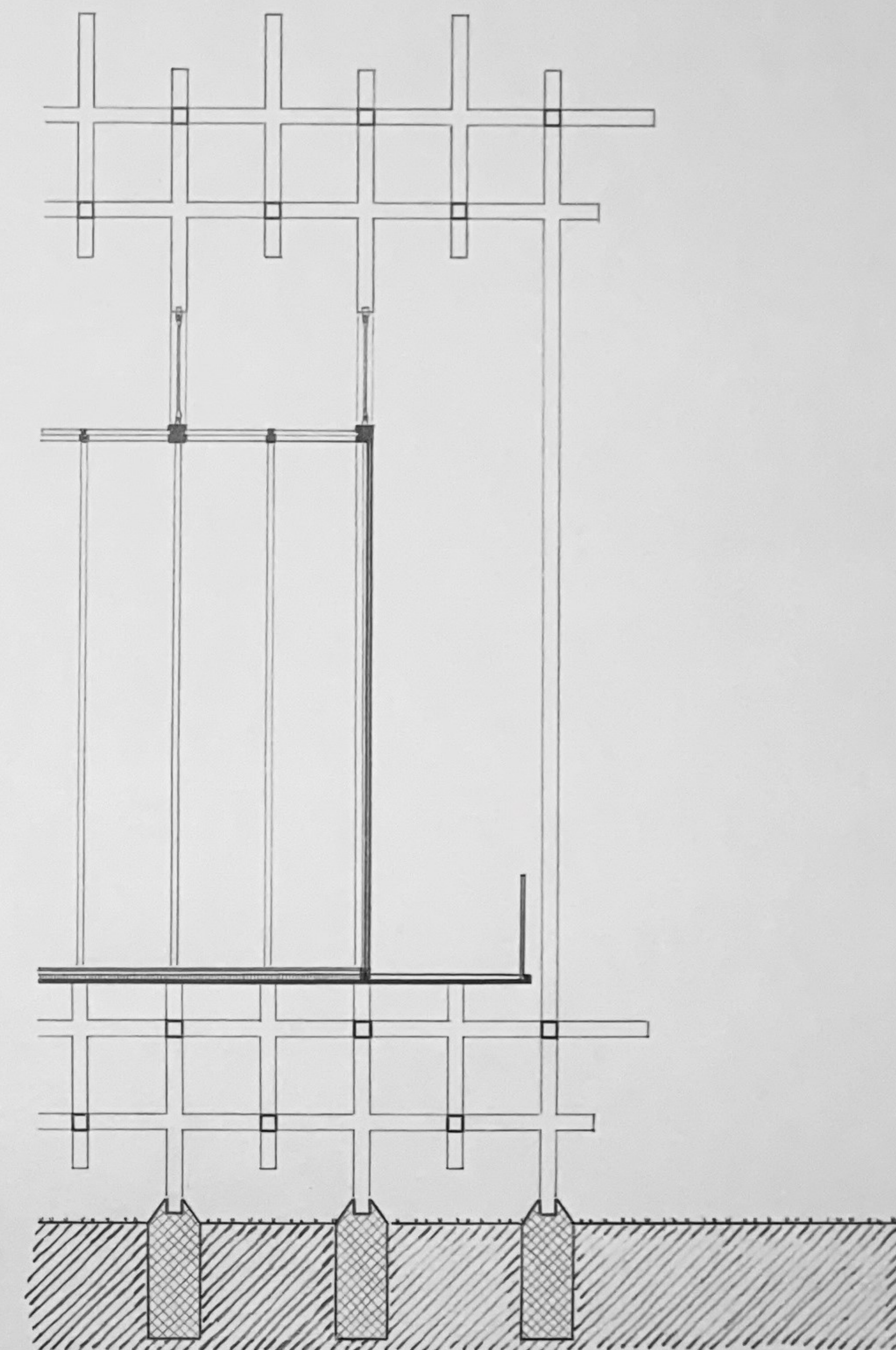
schnitt
