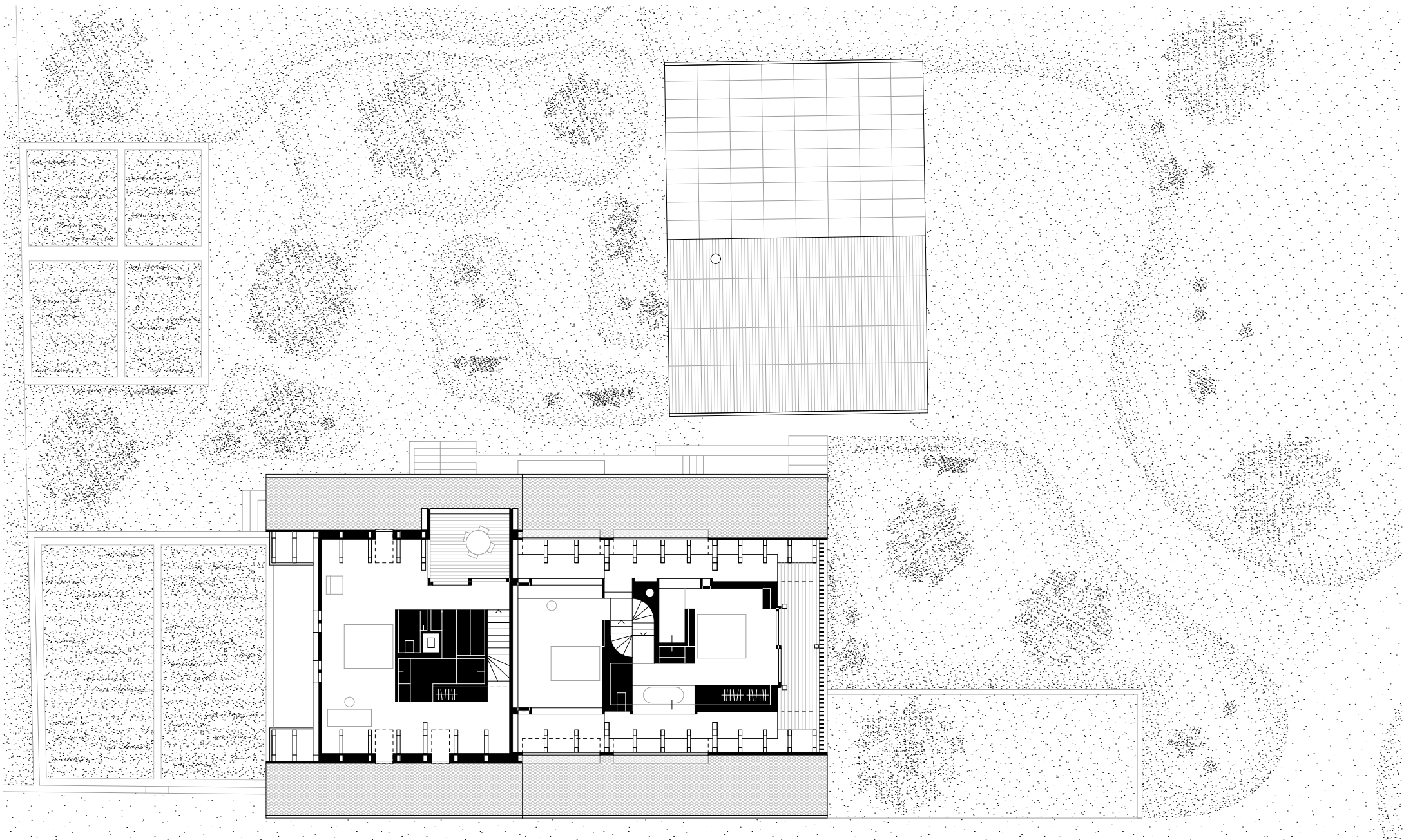
GRUNDRISS - DACHGESCHOSS
