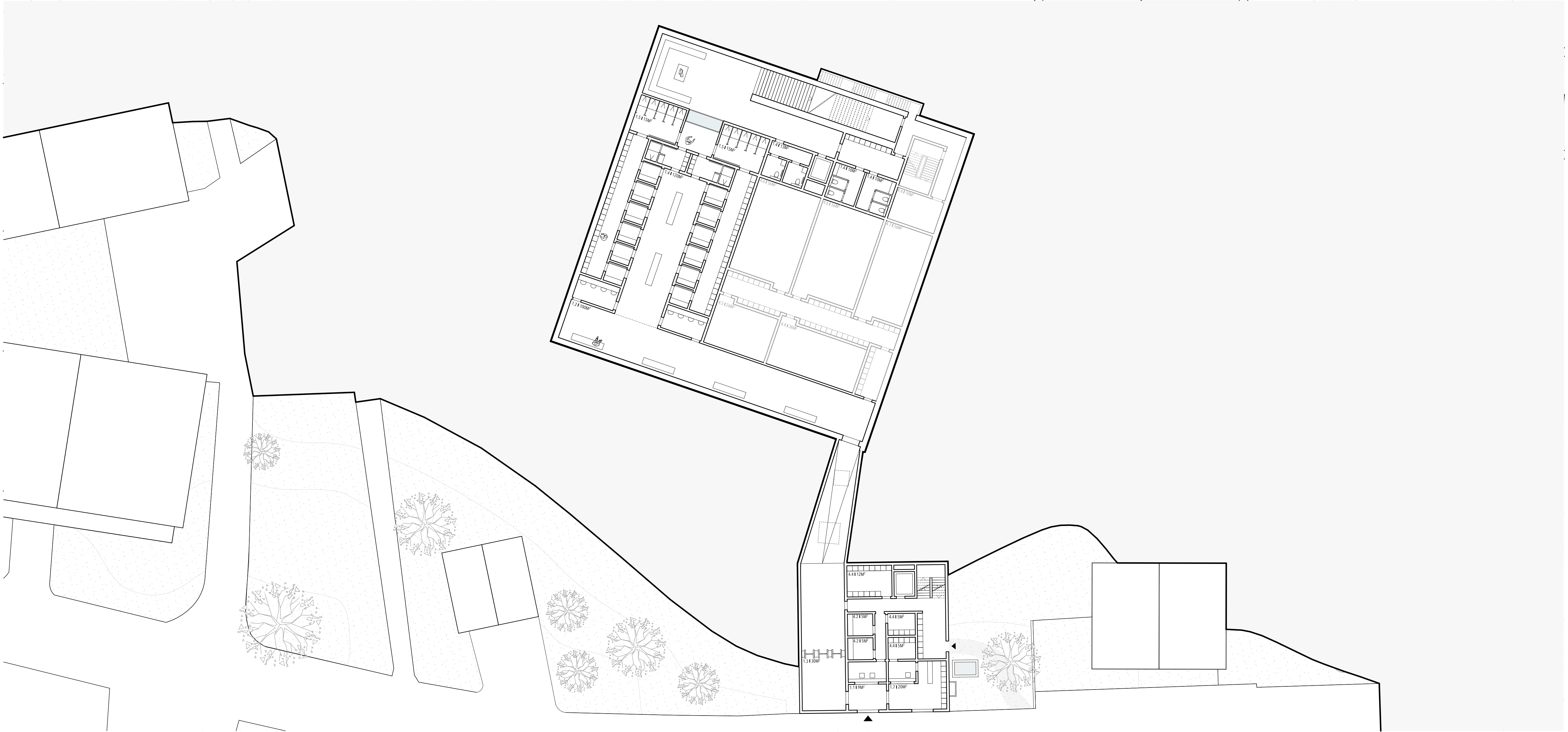
PLAN DU SOUS-SOL 1:200
