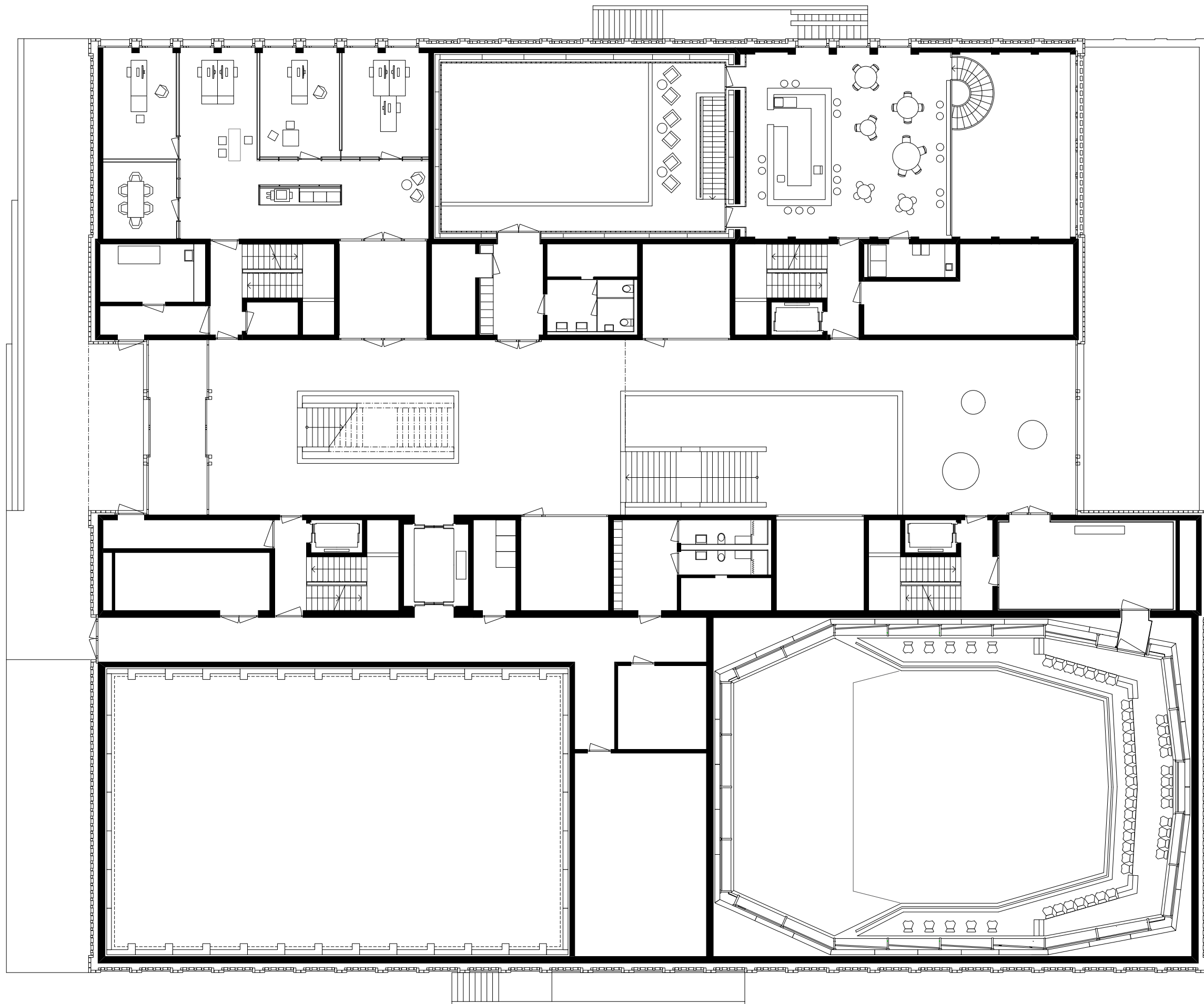
Grundriss EG Neubau Hochschule Luzern - Musik
